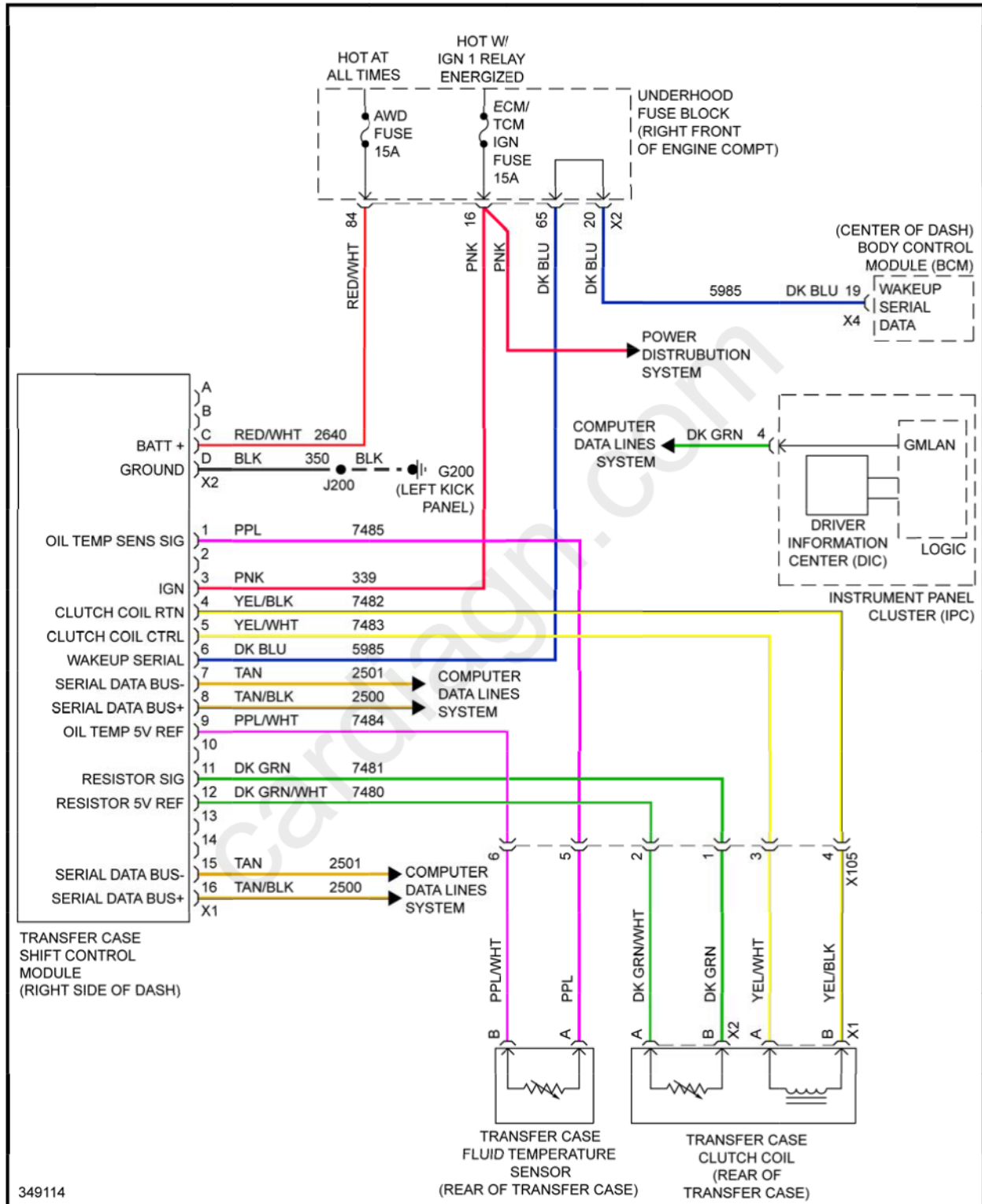
Fig. 116: AWD Circuit
