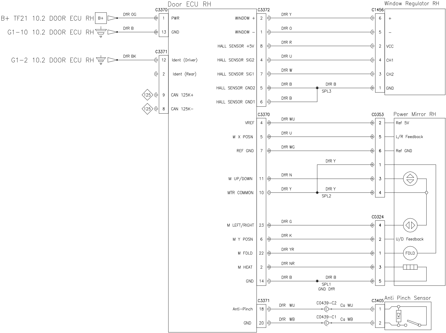
Door-Front Right LHD (Passenger Door Switchpack)
