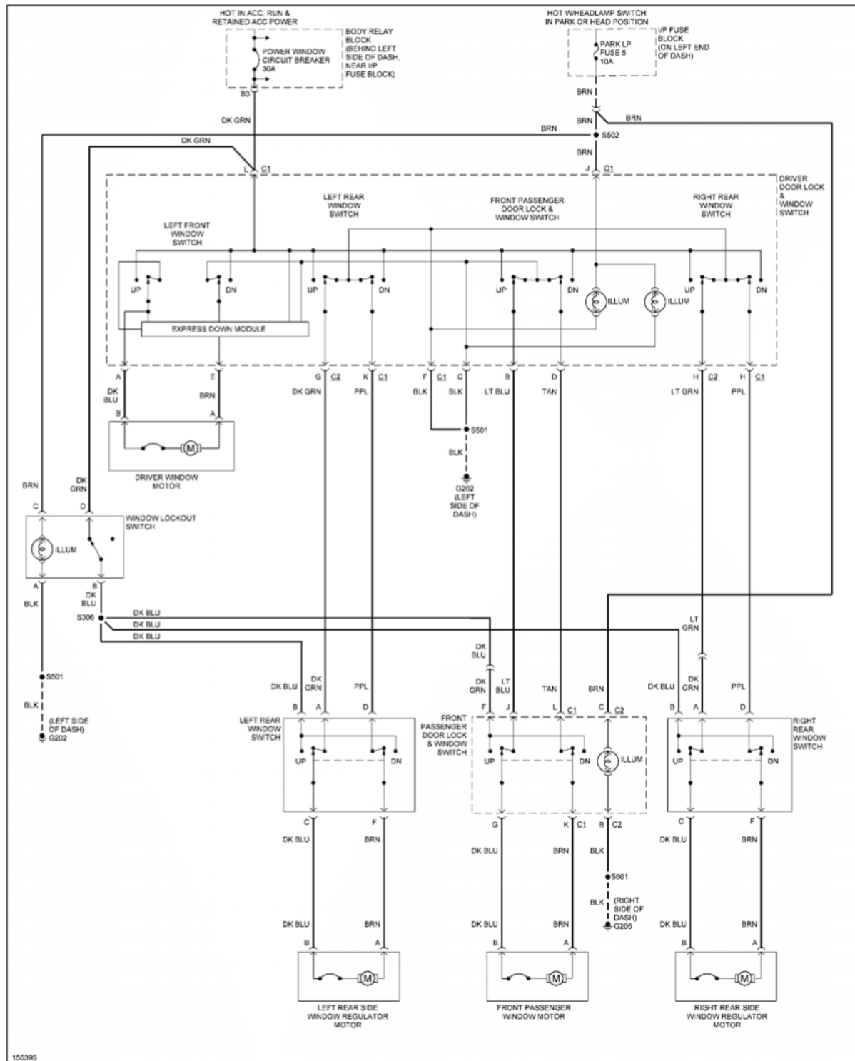
Fig. 43: Power Windows Circuit, 4 Door
