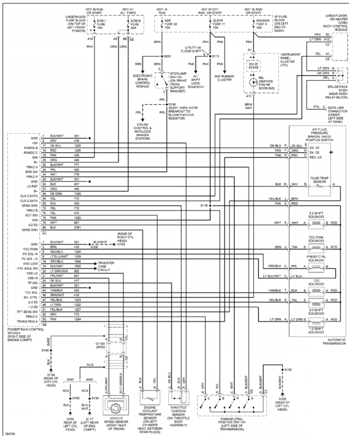
Fig. 51: A/T Circuit
