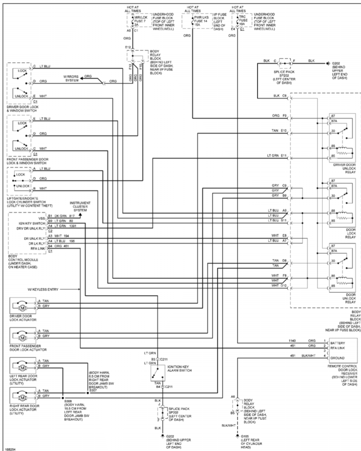
Fig. 33: Power Door Locks Circuit
