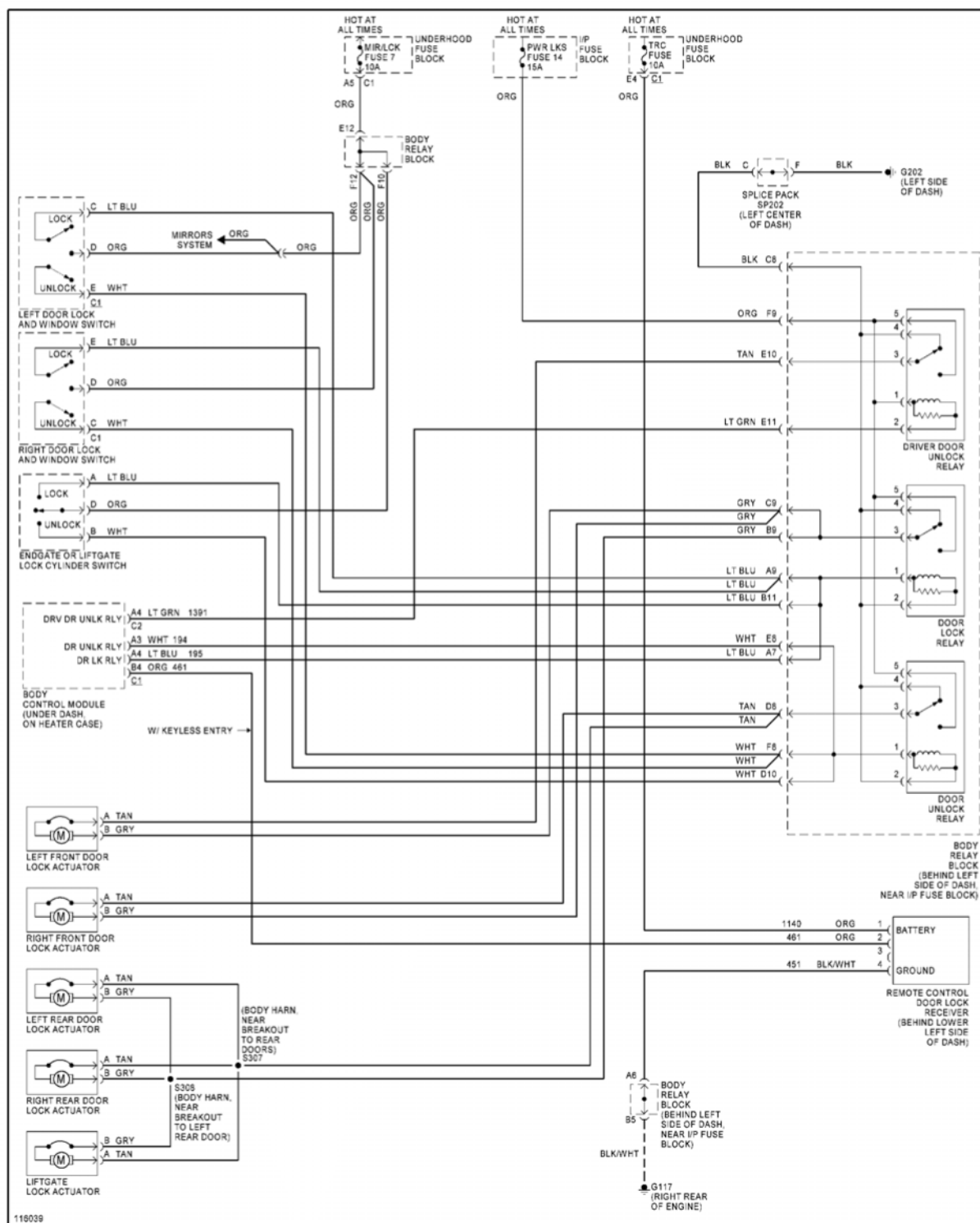
Fig. 35: Power Door Lock Circuit
