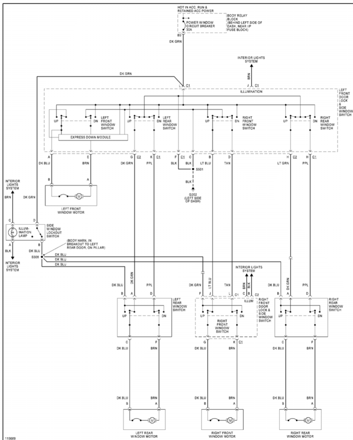
Fig. 43: Power Window Circuit, 4 Door
