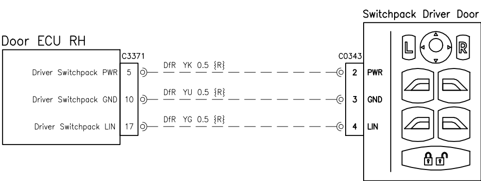
Door-Front Right RHD (Driver Door Switchpack)
