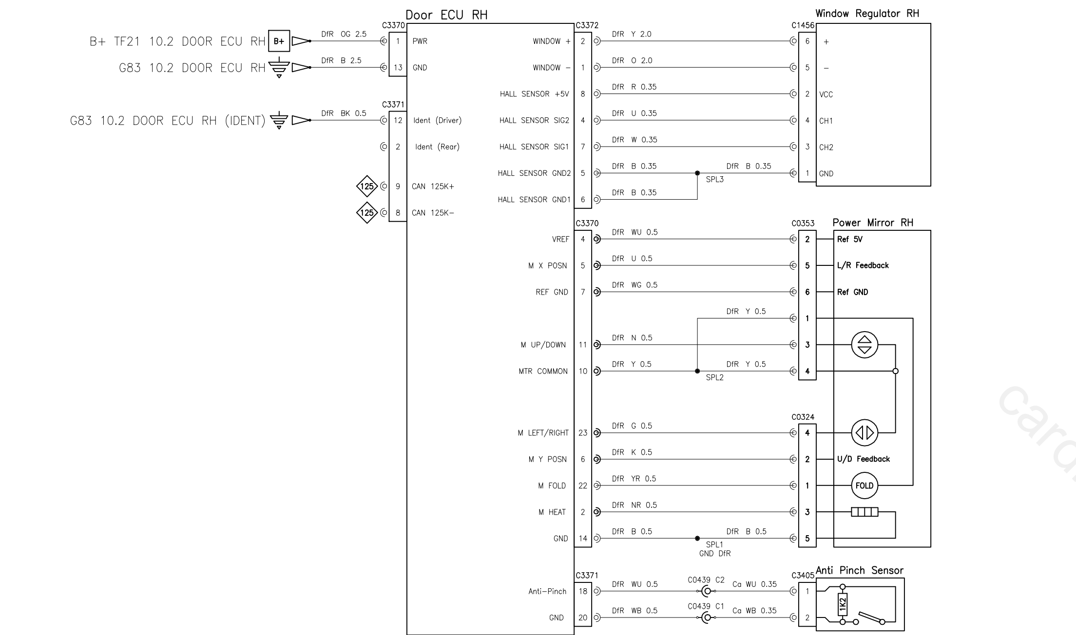
Door-Front Right LHD (Passenger Door Switchpack)
