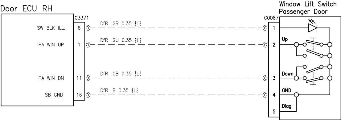
Door-Front Right LHD (Passenger Door Switchpack)
