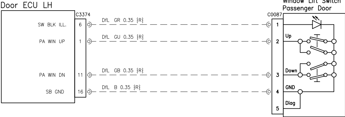
Door–Front Left RHD (Passenger Door Switchpack)
