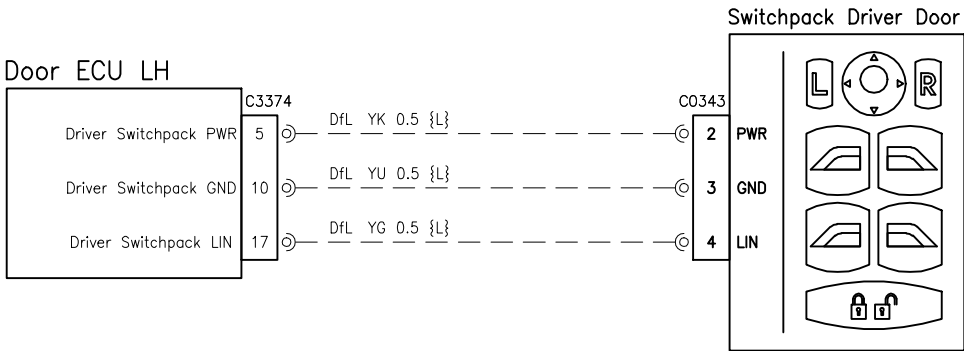
Door–Front Left LHD (Driver Door Switchpack)
