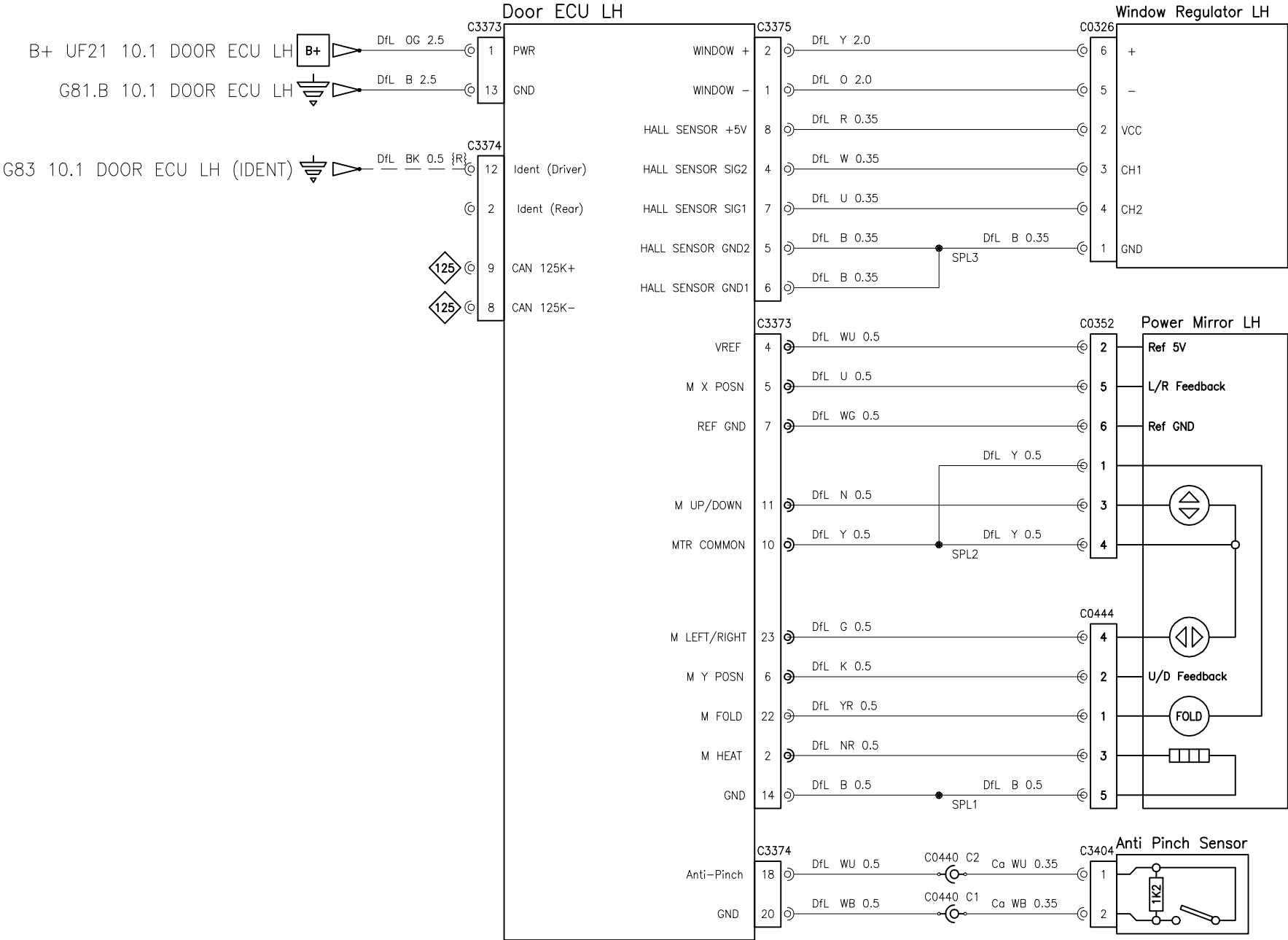
Door–Front Left LHD (Driver Door Switchpack)
