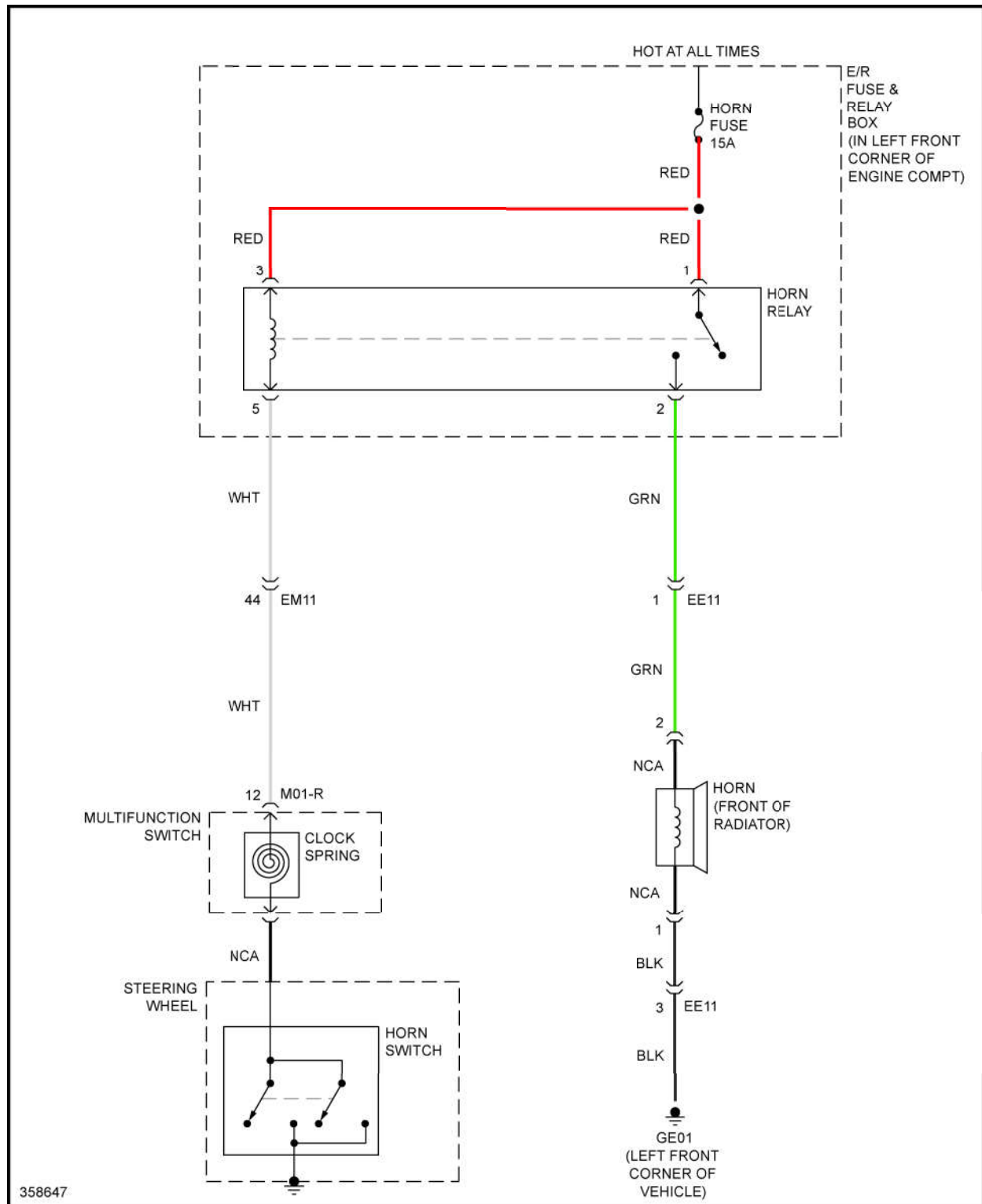
Fig. 37: Horn Circuit
