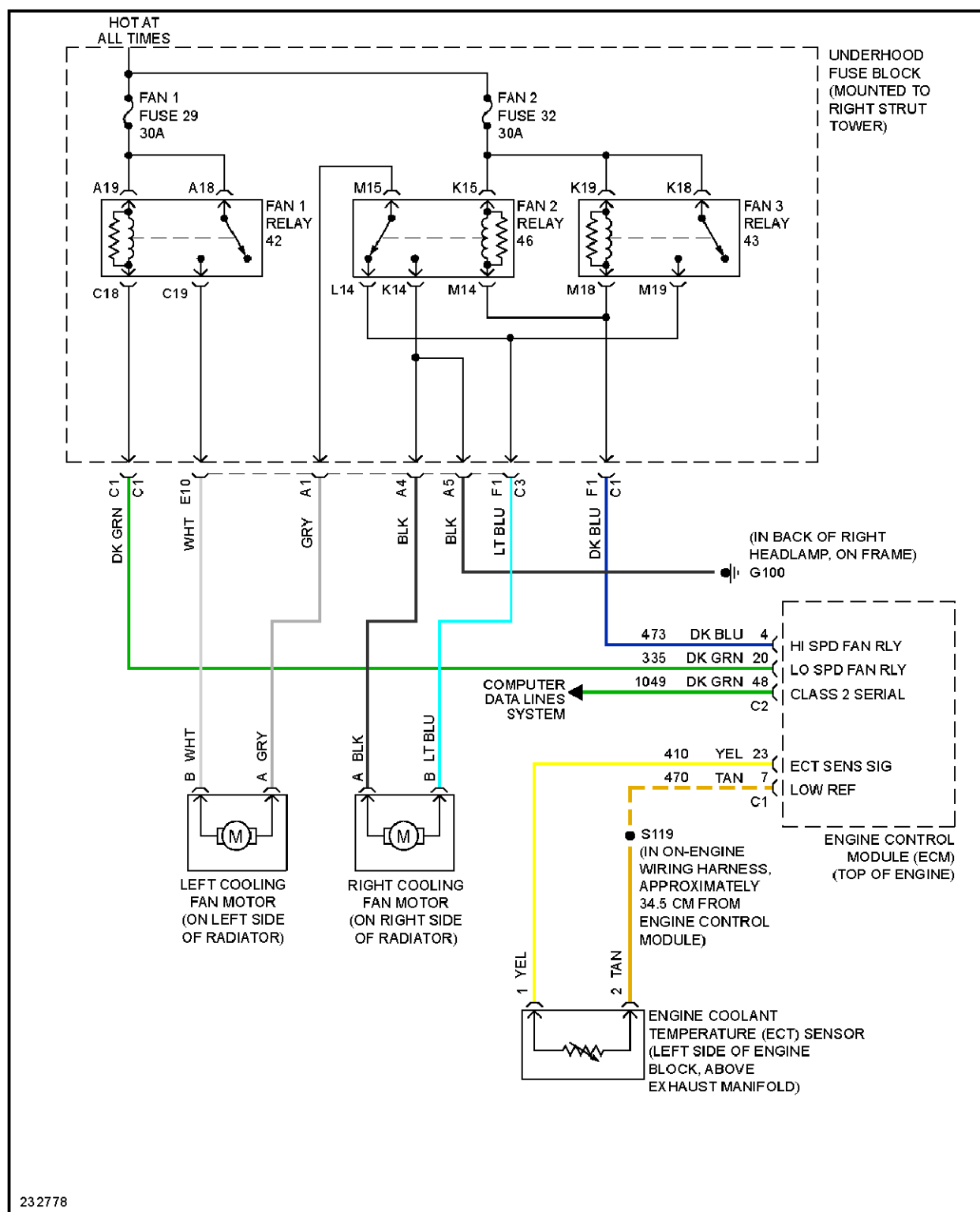
Fig. 14: 3.6L VIN 7, Cooling Fan Circuit
