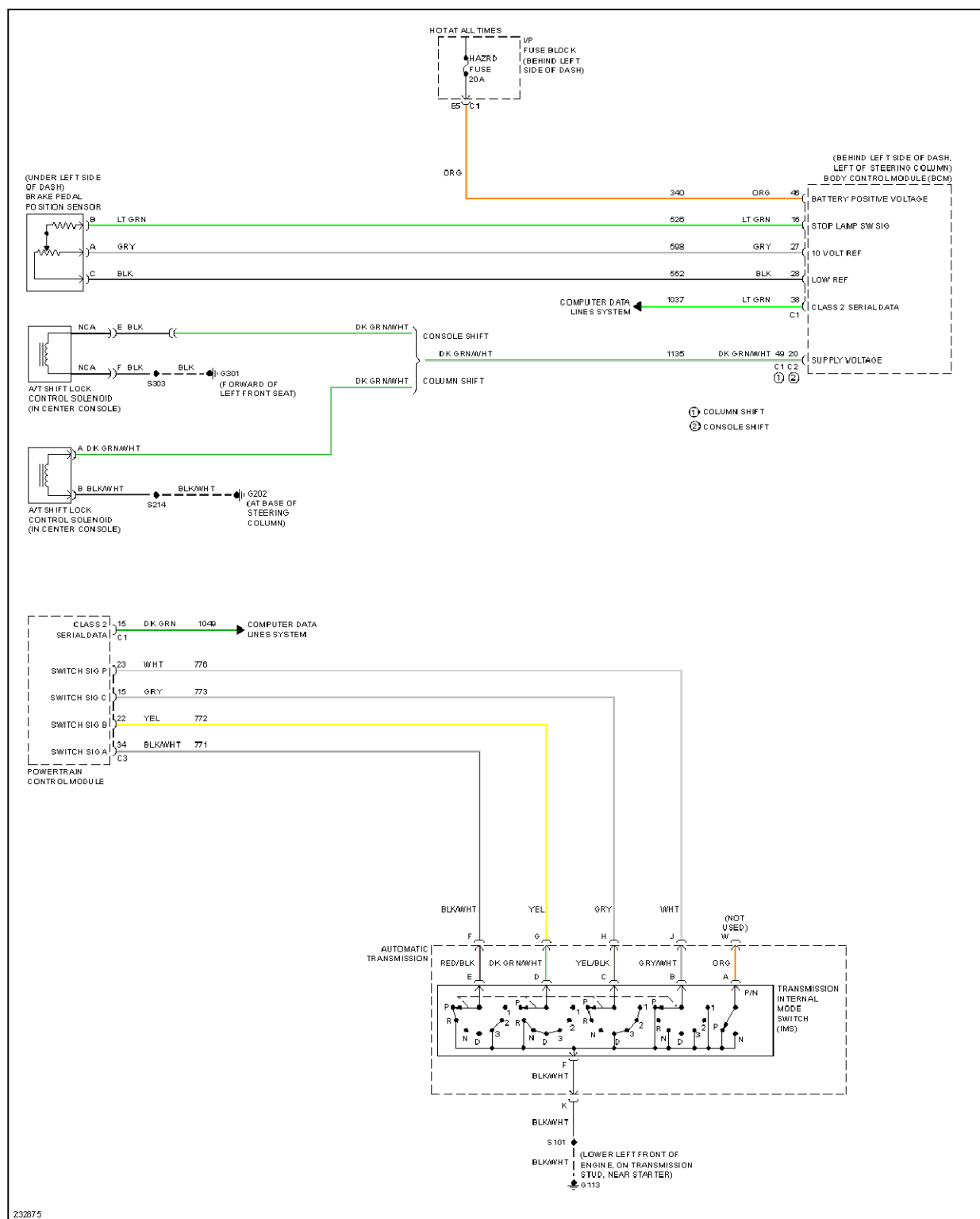
Fig. 62: 3.8L VIN 2, Shift Interlock Circuit
