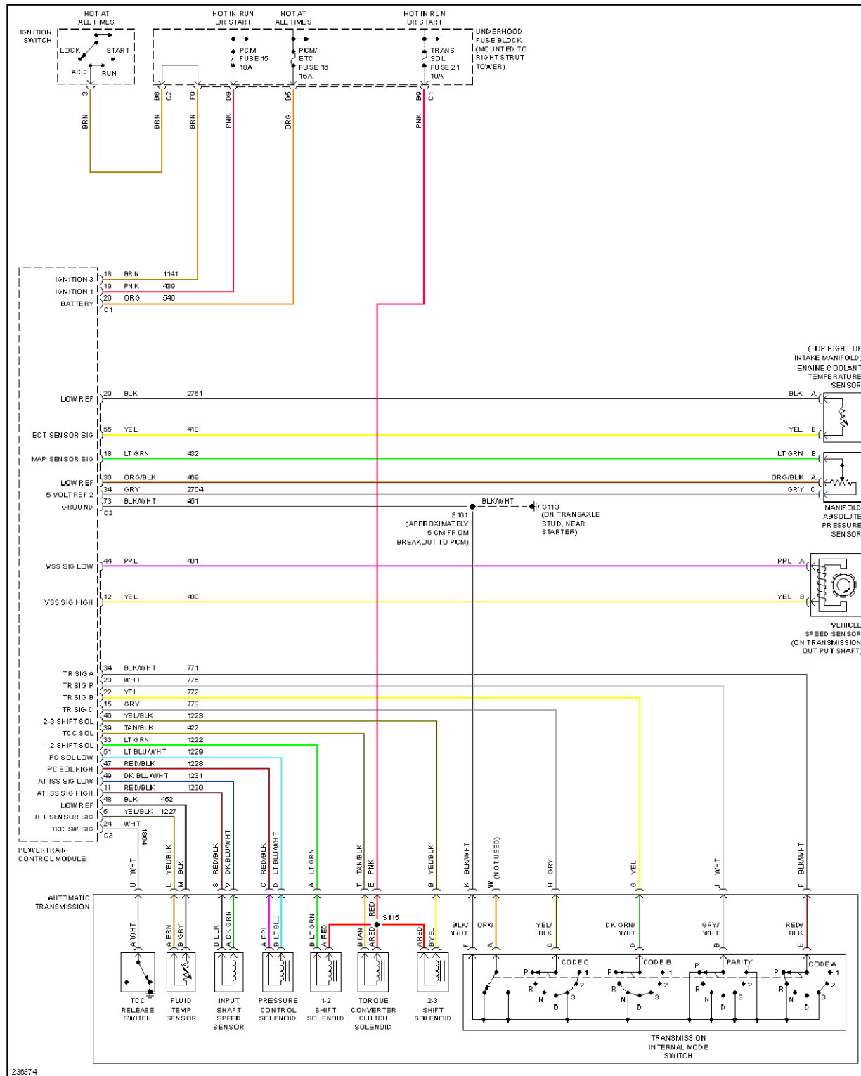
Fig. 68: 3.8L VIN 2, A/T Circuit
