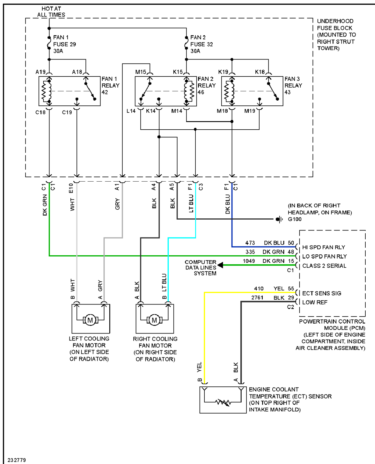
Fig. 15: 3.8L VIN 2, Cooling Fan Circuit
