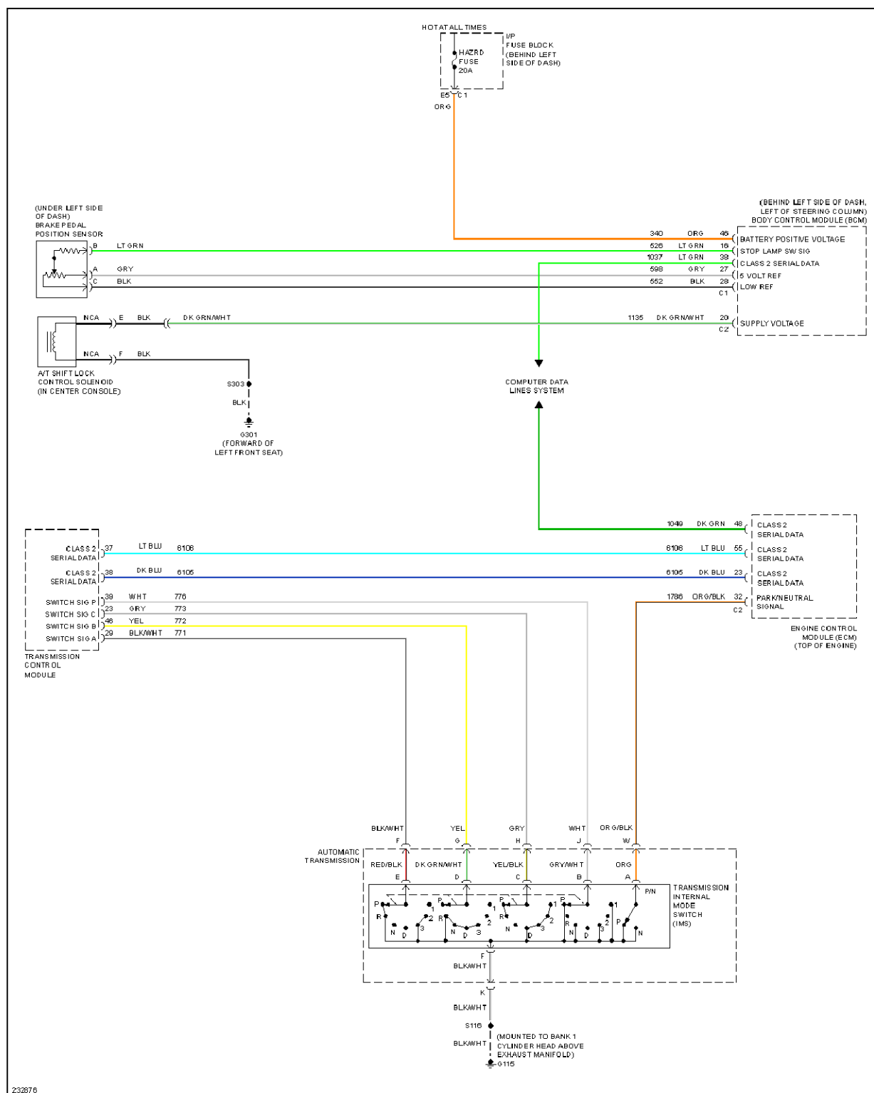
Fig. 61: 3.6L VIN 7, Shift Interlock Circuit
