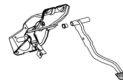
50100 制动踏板 Brake Pedal
