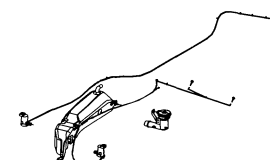
61800 洗涤器总成 Washer Assembly
