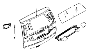
70500 后背门总成 Tailgate Assembly
