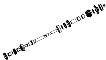
30100 前驱动桥总成 Front Drive Axle Assembly
