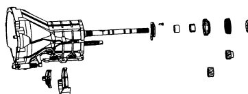
20700 接箱组件 Gearbox Assembly
