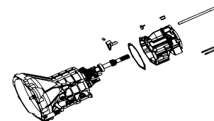
20900 变速器带分动器操纵杆总成 Controller Cover Assembly
