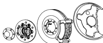
50300 前制动器总成 Front Brake Assembly
