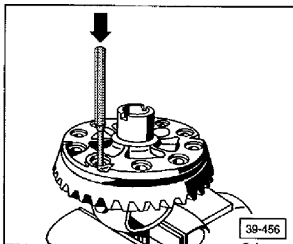
► Fig. 4 Ring gear, removing
