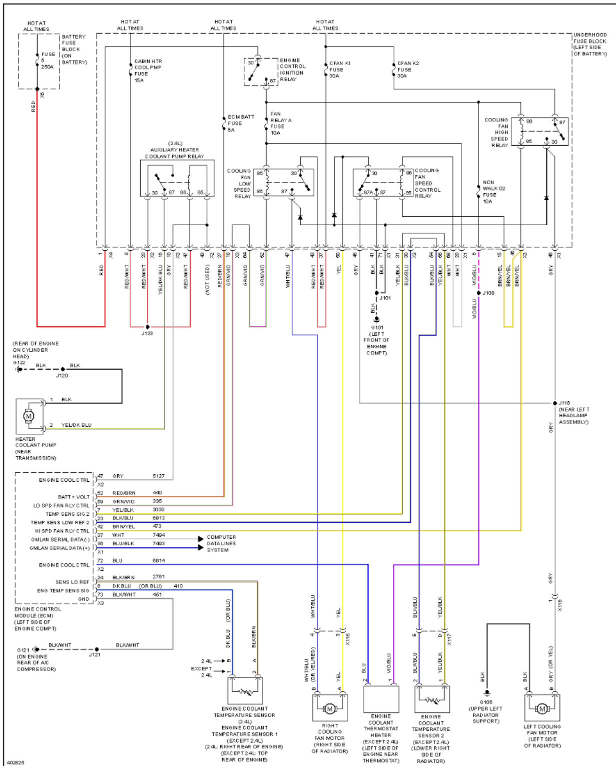
Fig. 24: Cooling Fan Circuit
