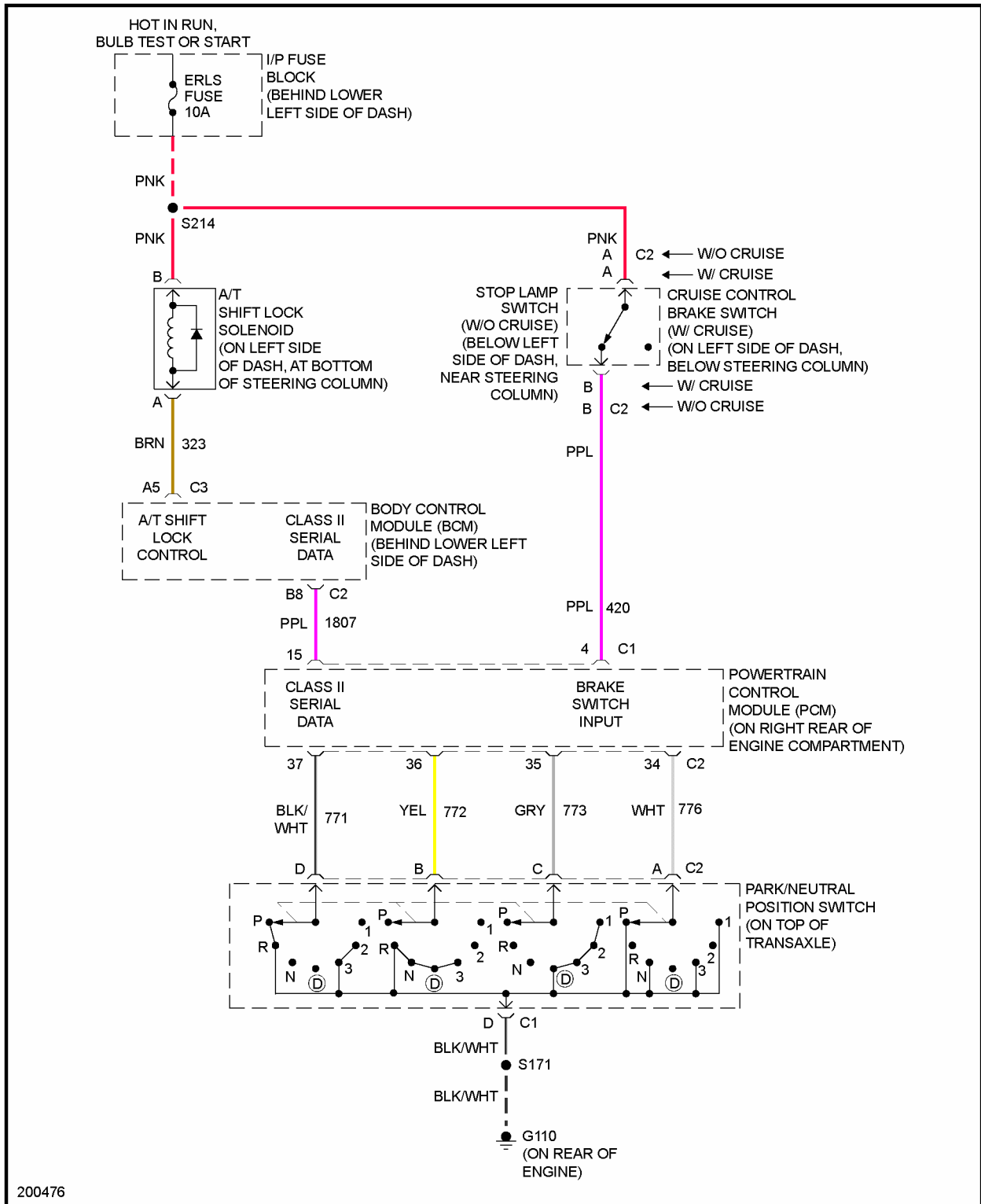
Fig. 35: Shift Interlock Circuit
