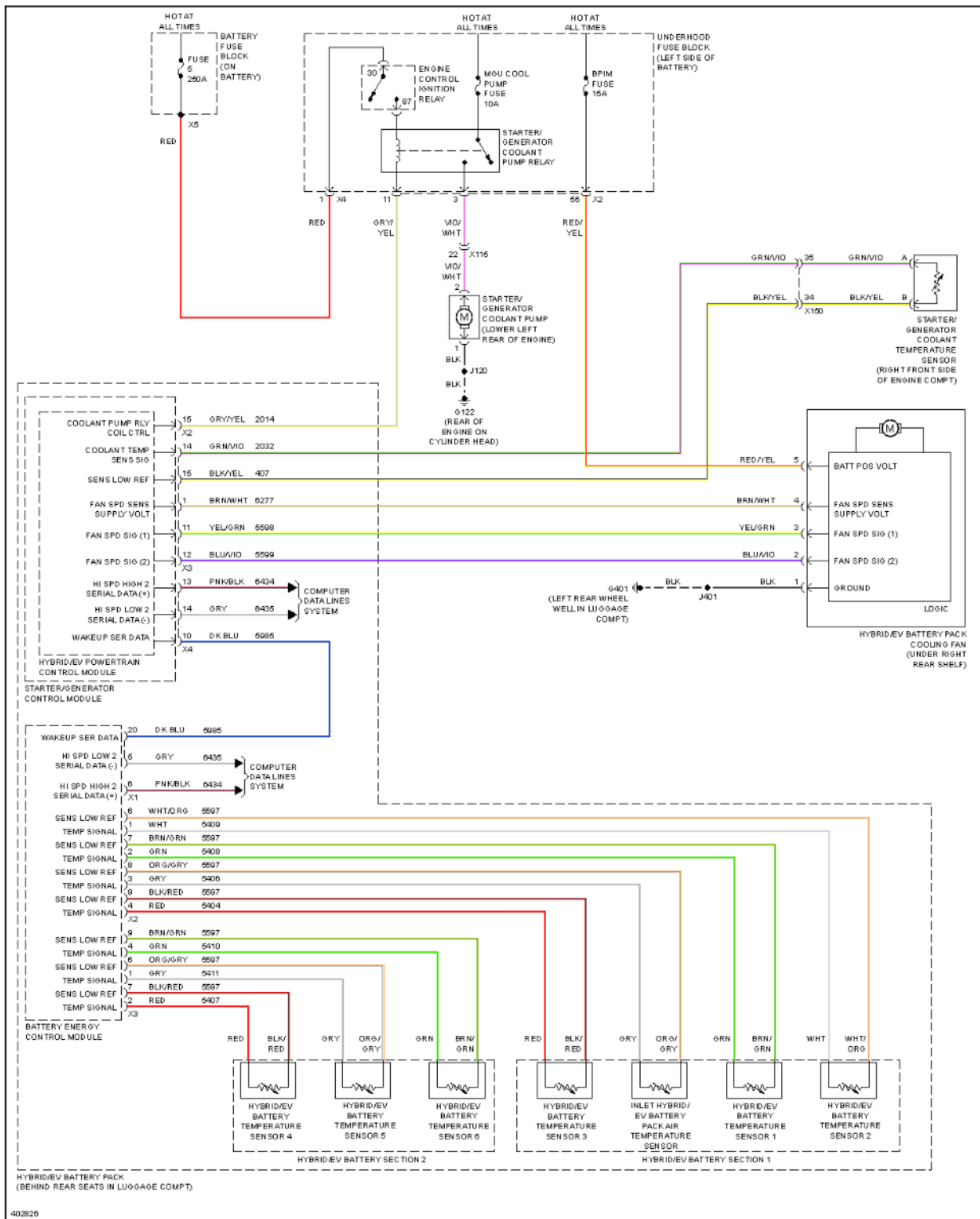
Fig. 25: Hybrid Cooling Fan Circuit
