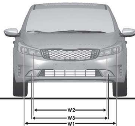
<Расстояние между лампами фар>
