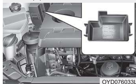
■ Панель с предохранителями в моторном отсеке (дизельный двигатель, со стороны пассажира)
