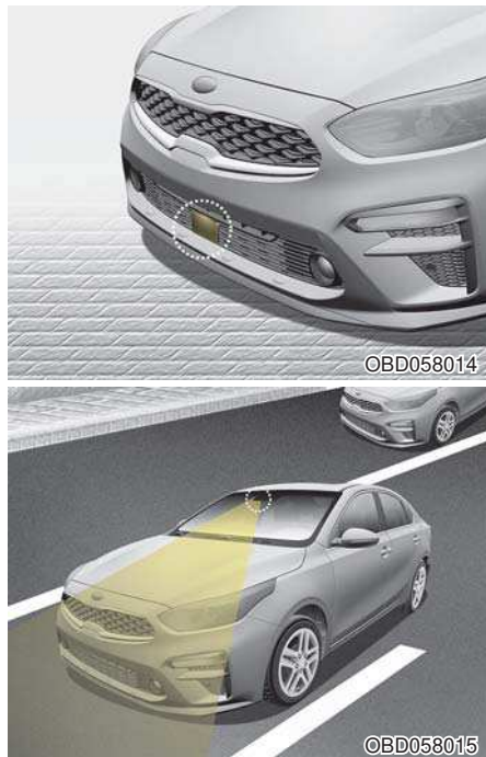
■ 차간거리 감지 센서(전방 레이더/전방 카메라) 전방의 차량을 감지하여 차간거리를 유지시켜 주는 센서입니다.
