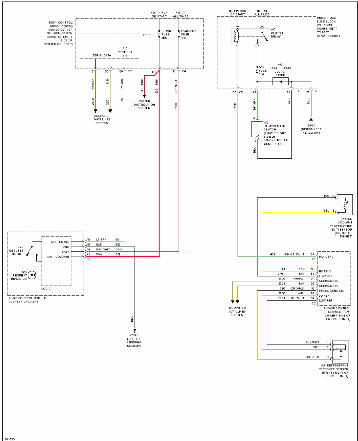
Fig. 4: 2.2L VIN F, Compressor Circuit
