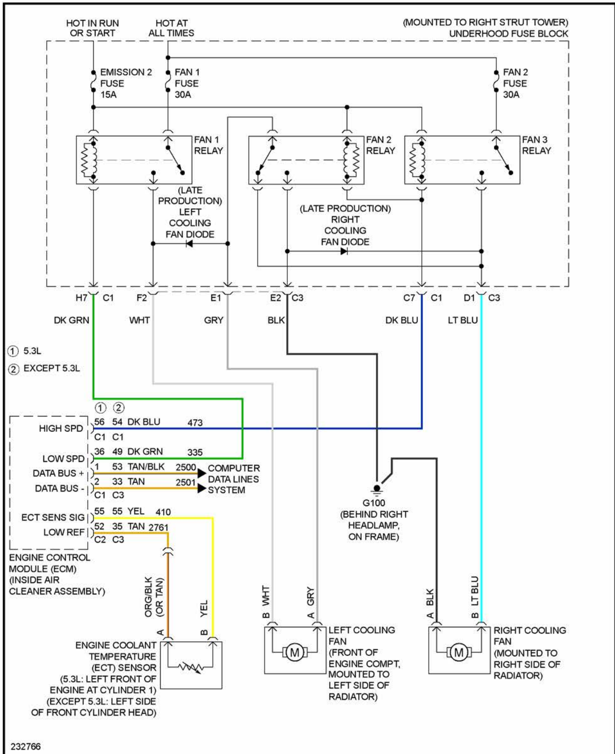
Fig. 12: Cooling Fan Circuit
