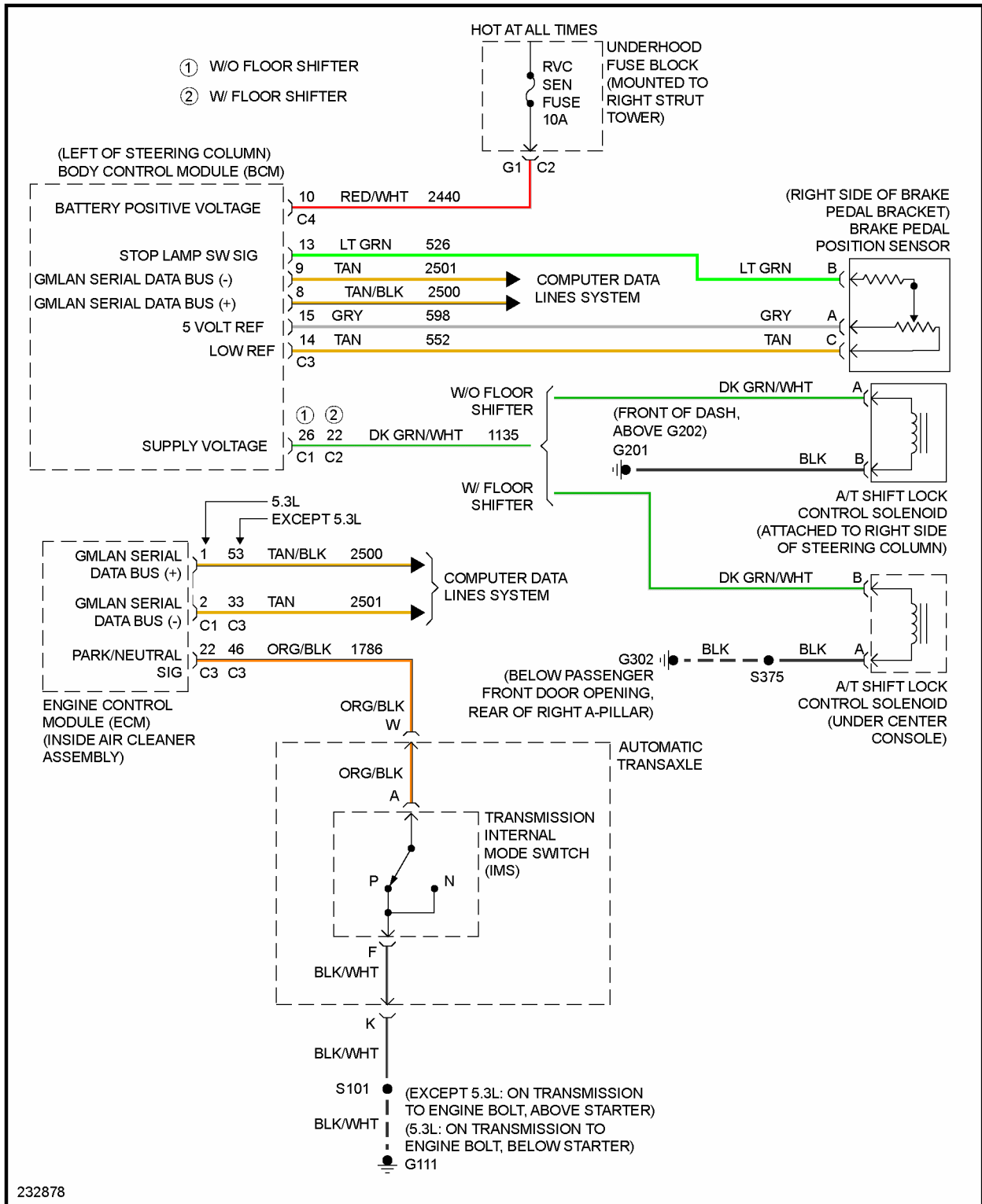
Fig. 58: Shift Interlock Circuit
