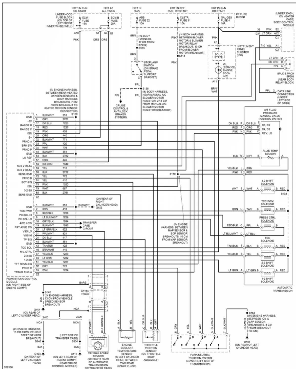
Fig. 51: A/T Circuit
