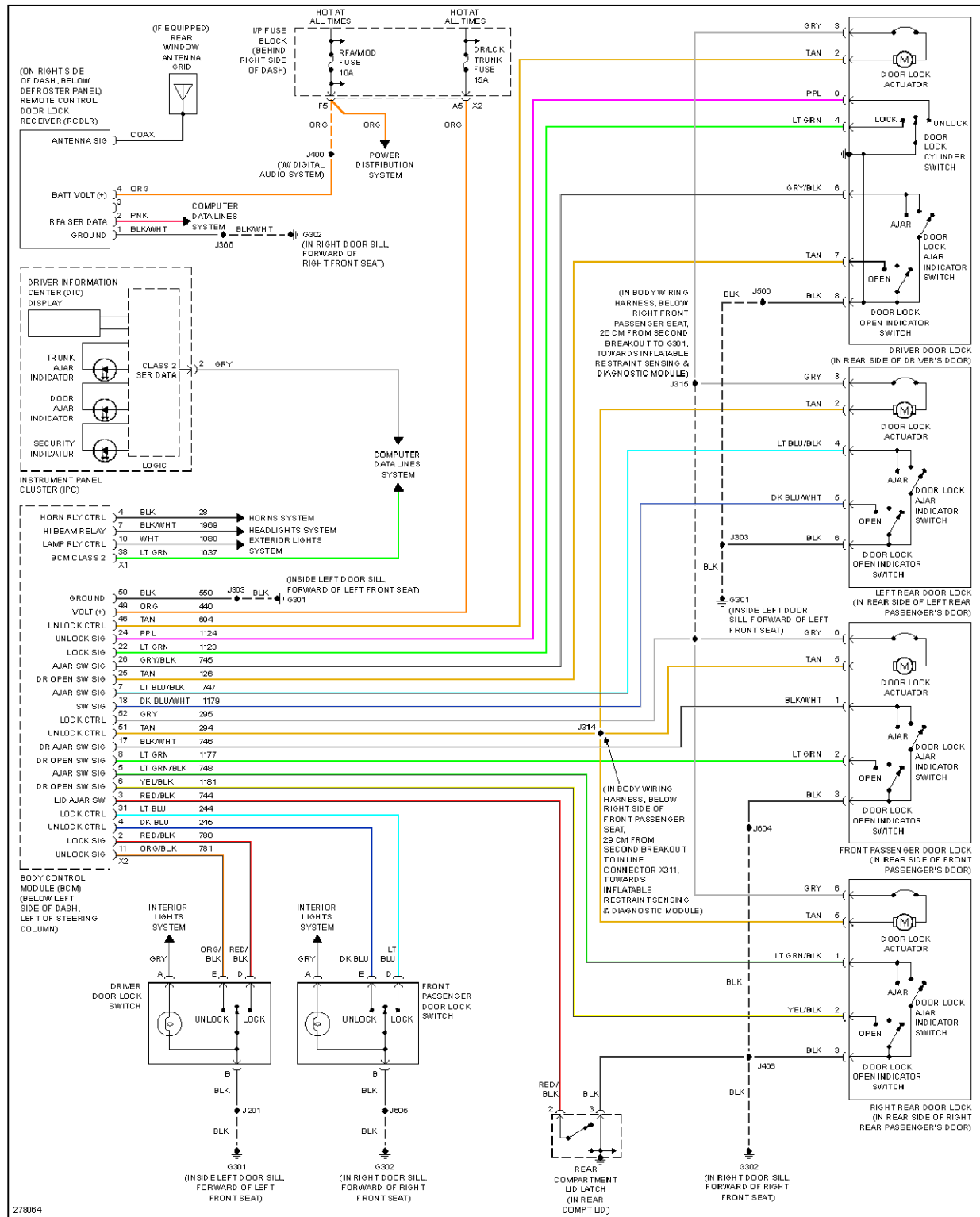
Fig. 67: Power Door Locks Circuit
