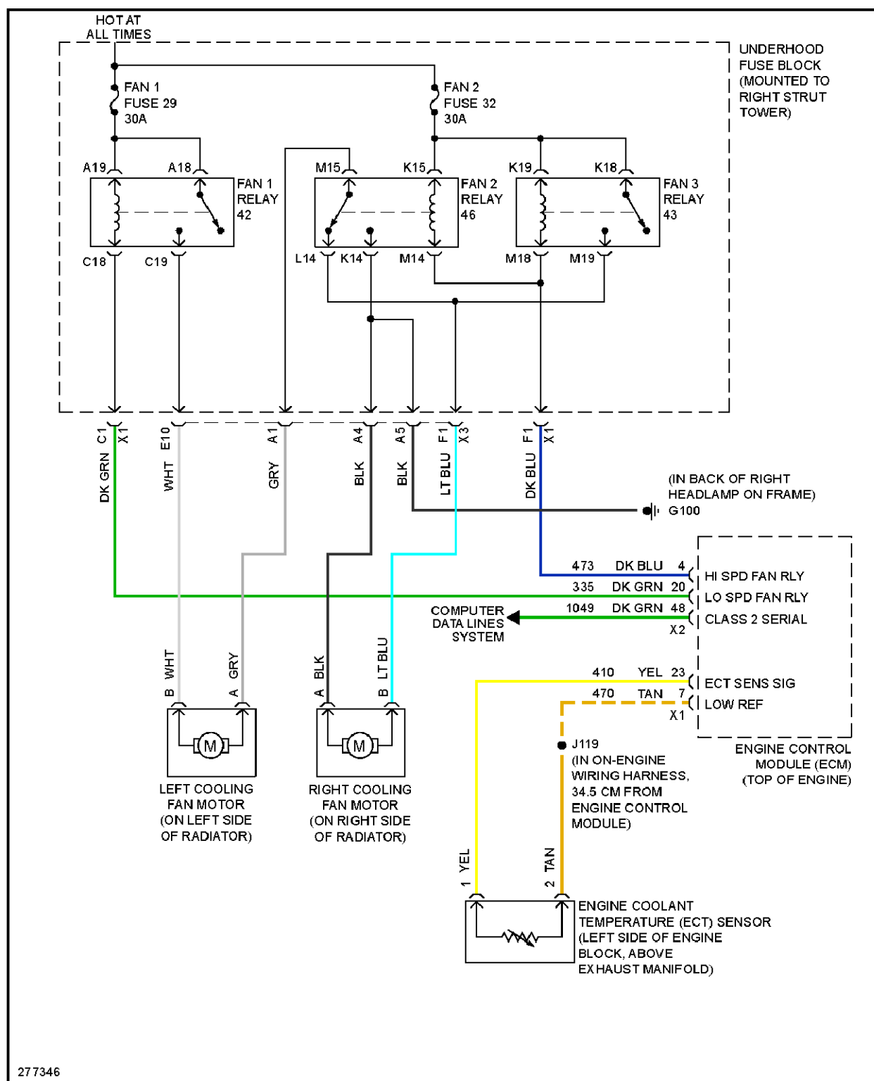
Fig. 16: 3.6L VIN 7, Cooling Fan Circuit
