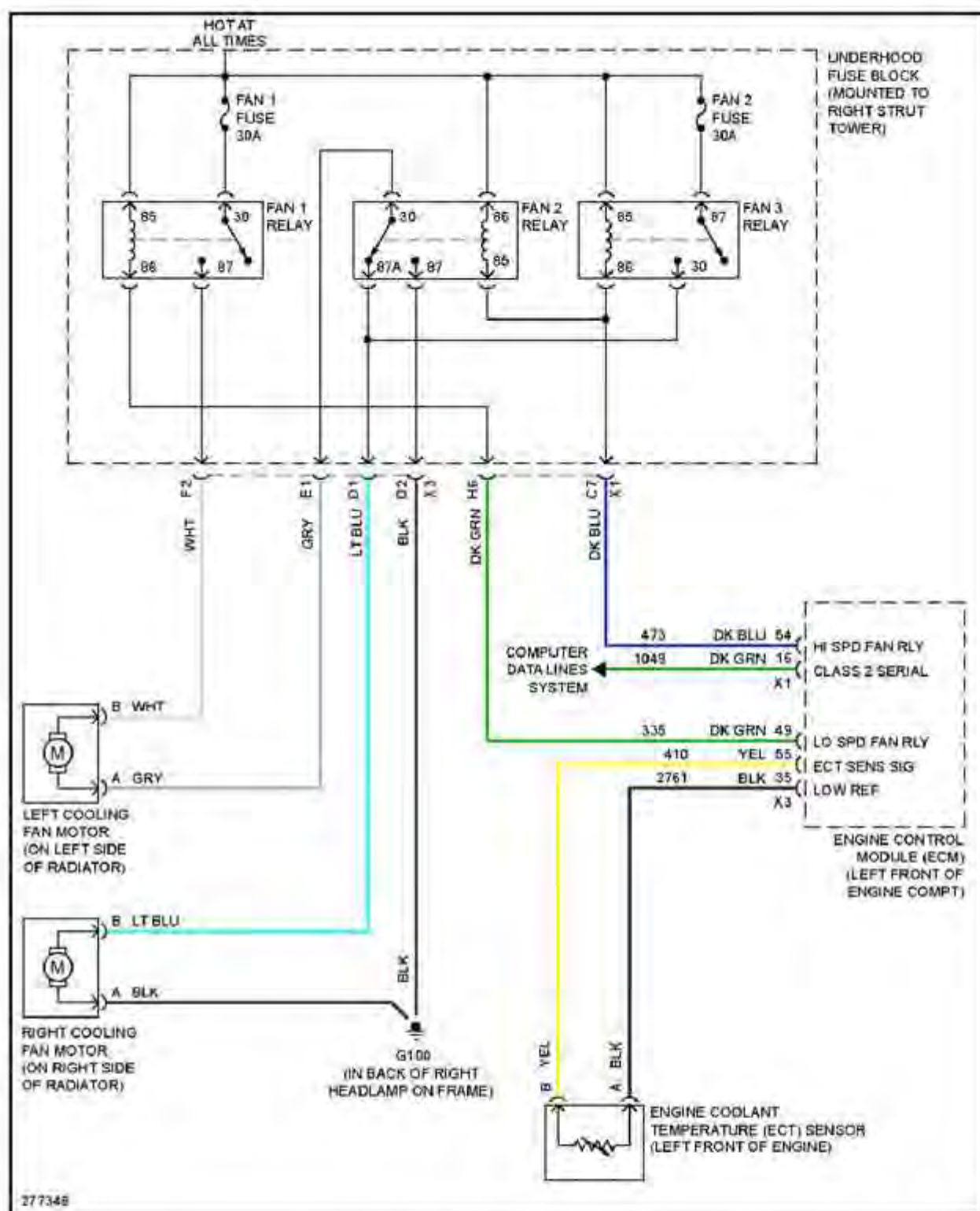
Fig. 18: 5.3L VIN C, Cooling Fan Circuit
