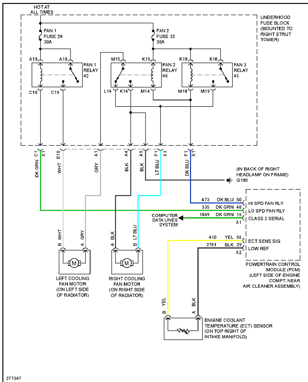
Fig. 17: 3.8L VIN 2, Cooling Fan Circuit
