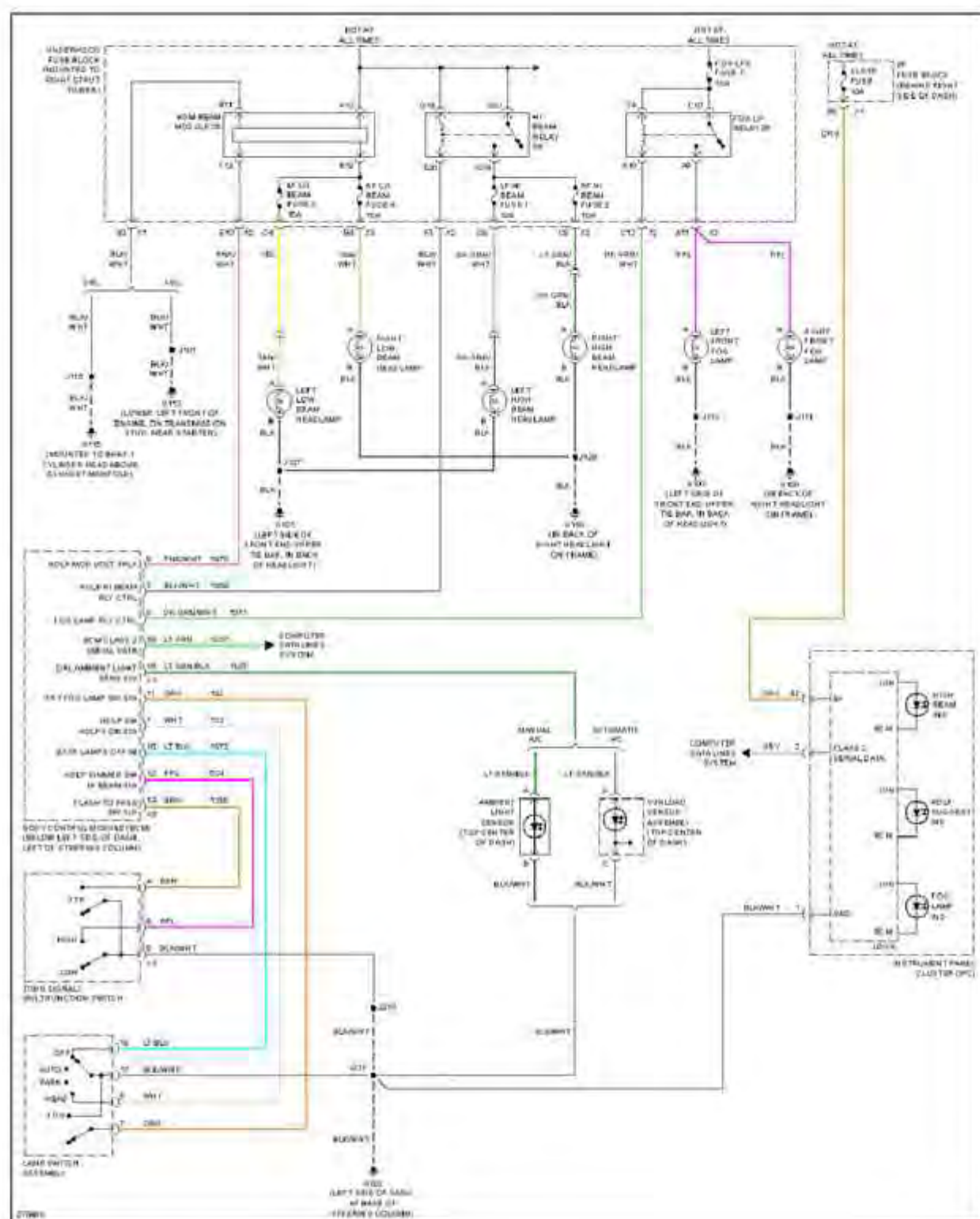
Fig. 46: 3.8L VIN 2, Headlights Circuit
