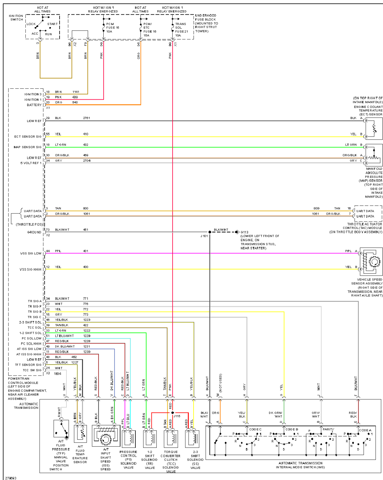
Fig. 90: 3.8L VIN 2, Transmission Circuit
