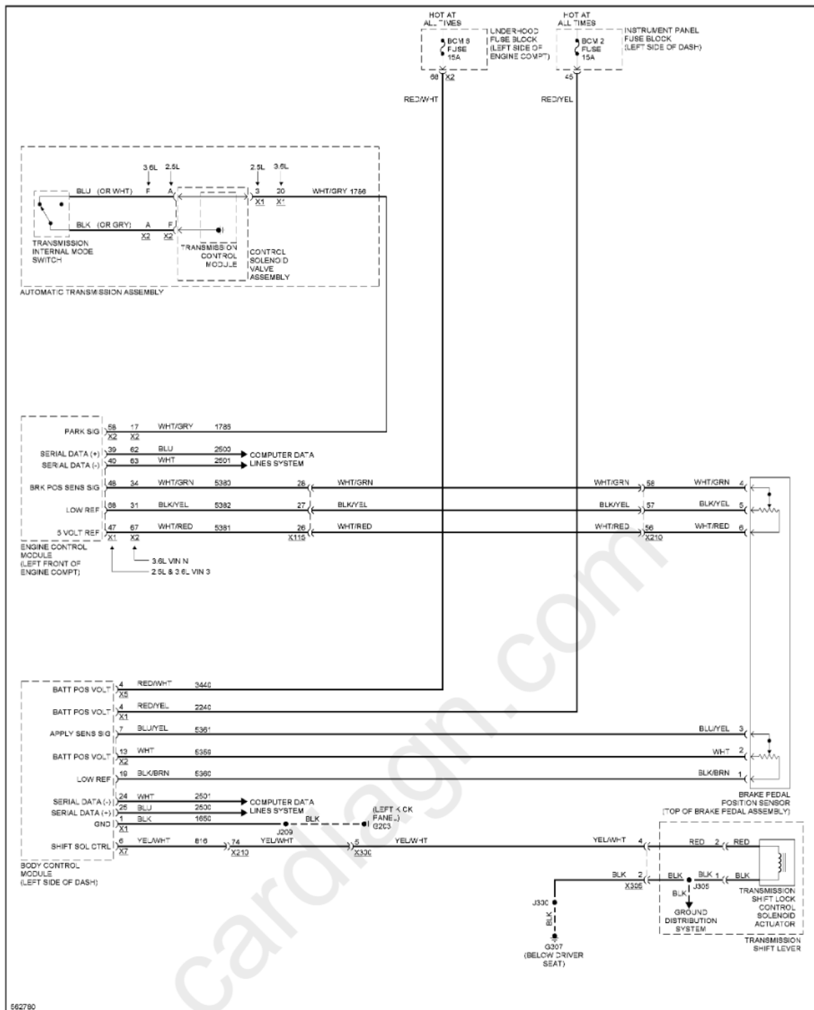
Fig. 117: Shift Interlock Circuit
