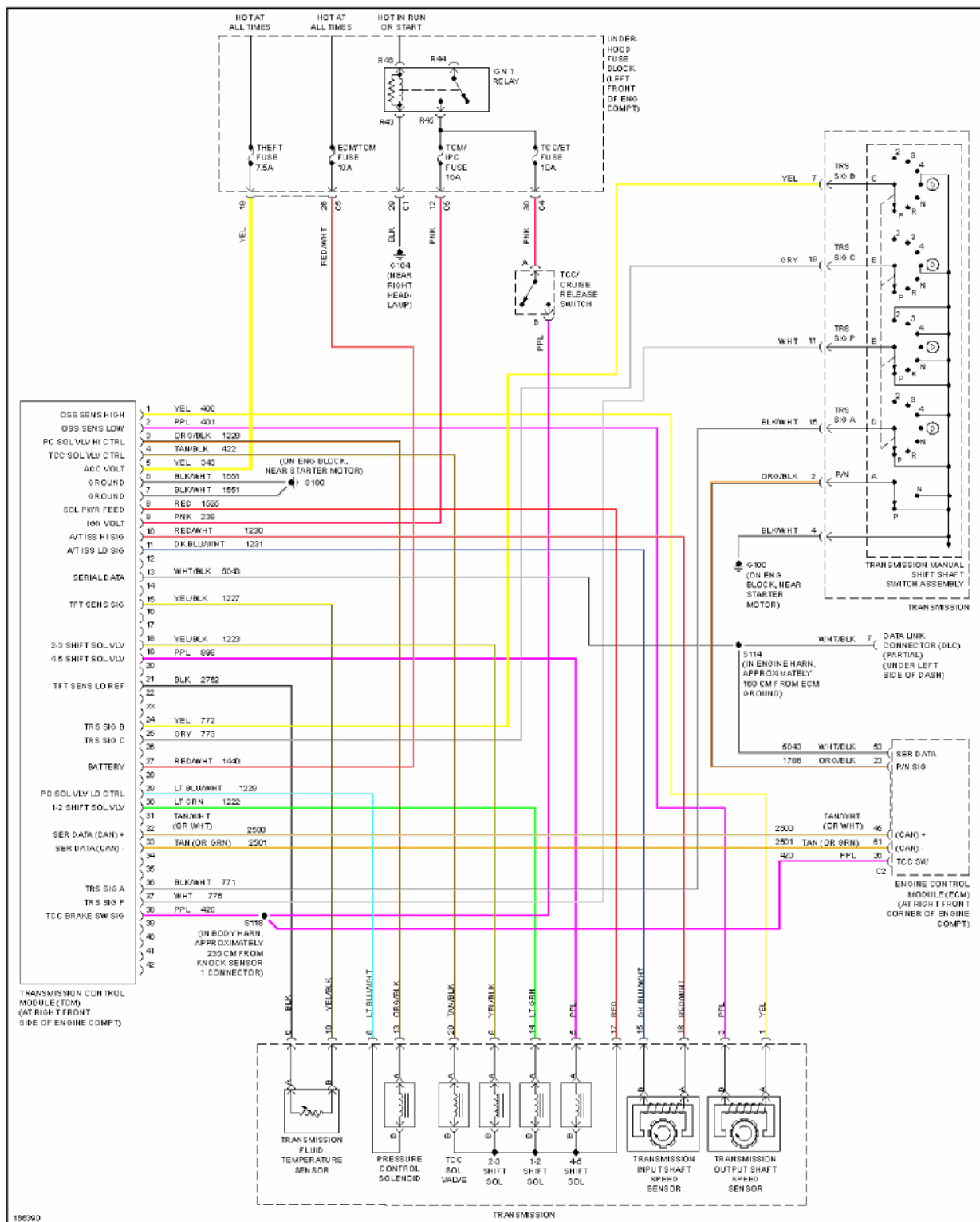
Fig. 65: 3.2L VIN N, A/T Circuit
