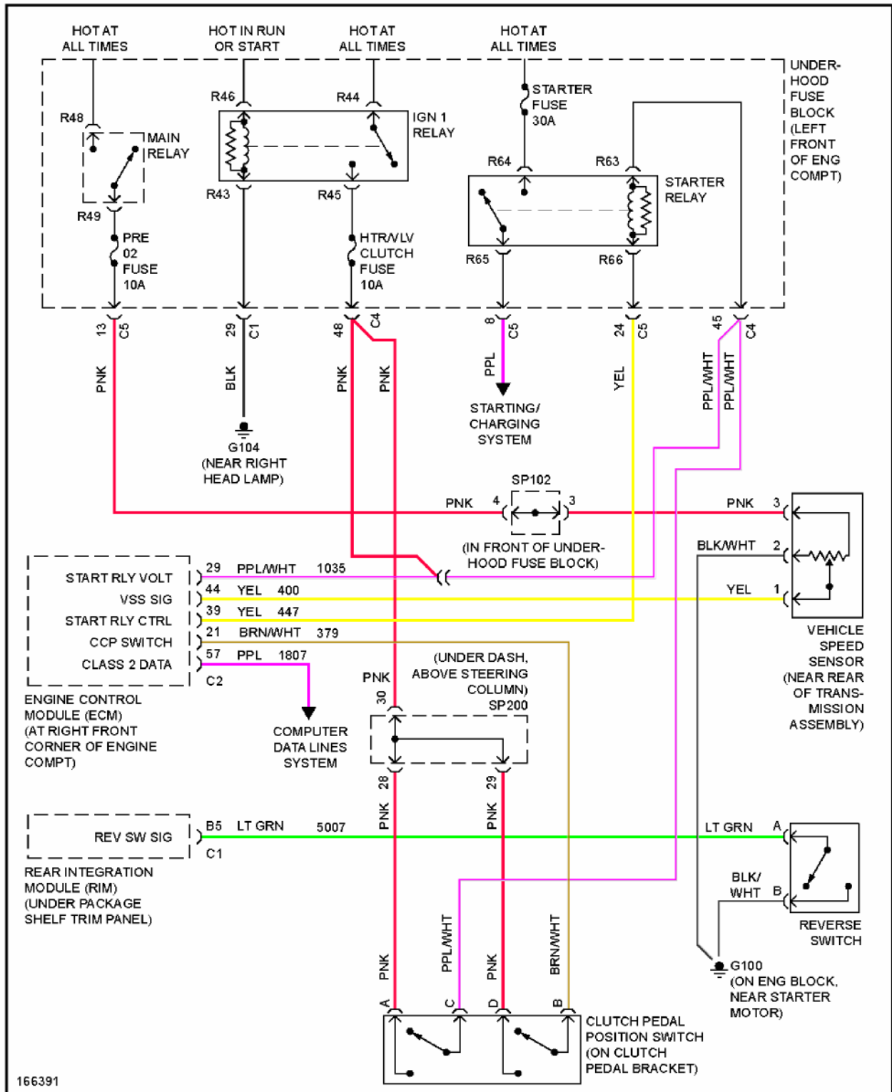
Fig. 66: 3.2L VIN N, M/T Circuit
