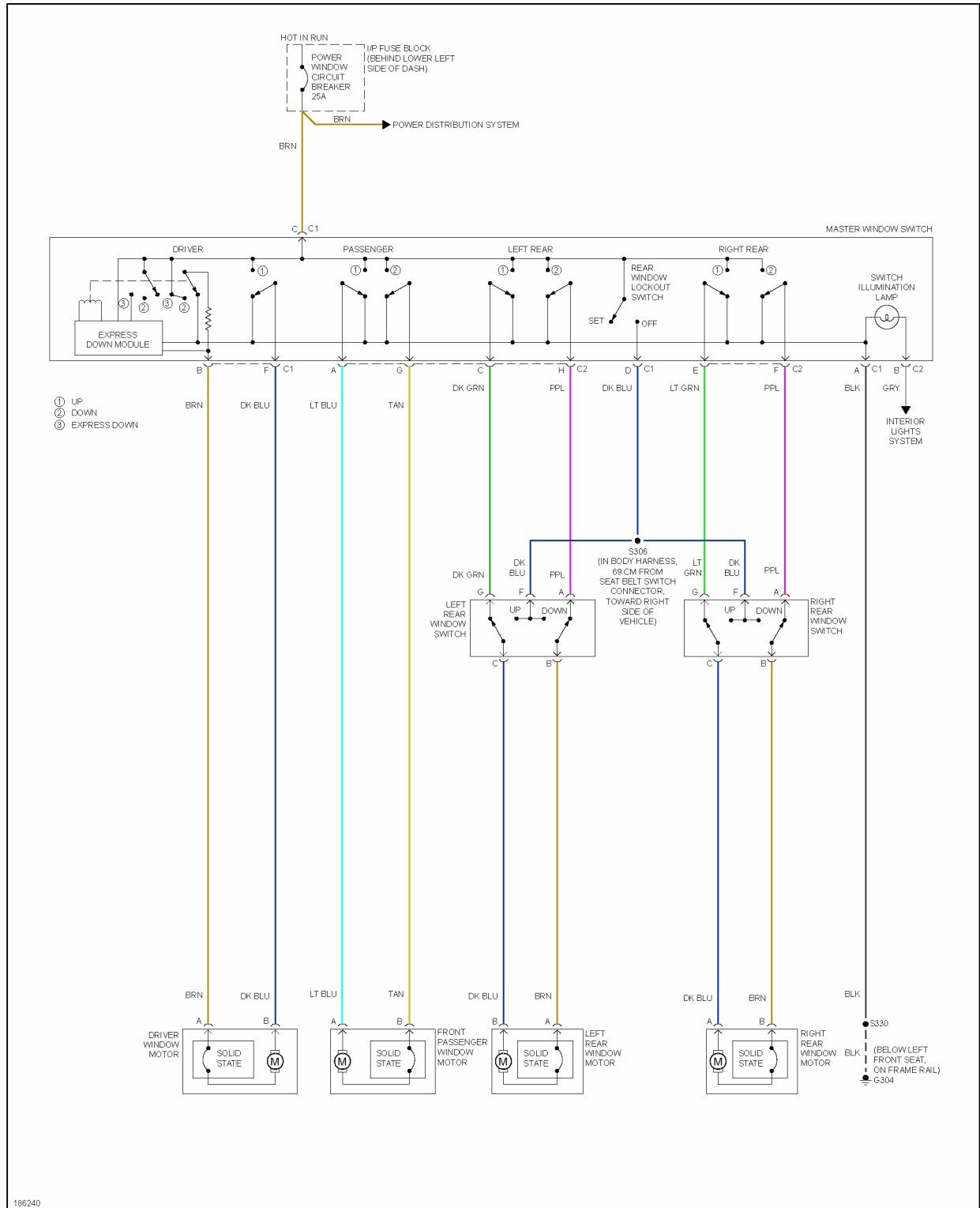
Fig. 29: Power Windows Circuit, 4 Door
