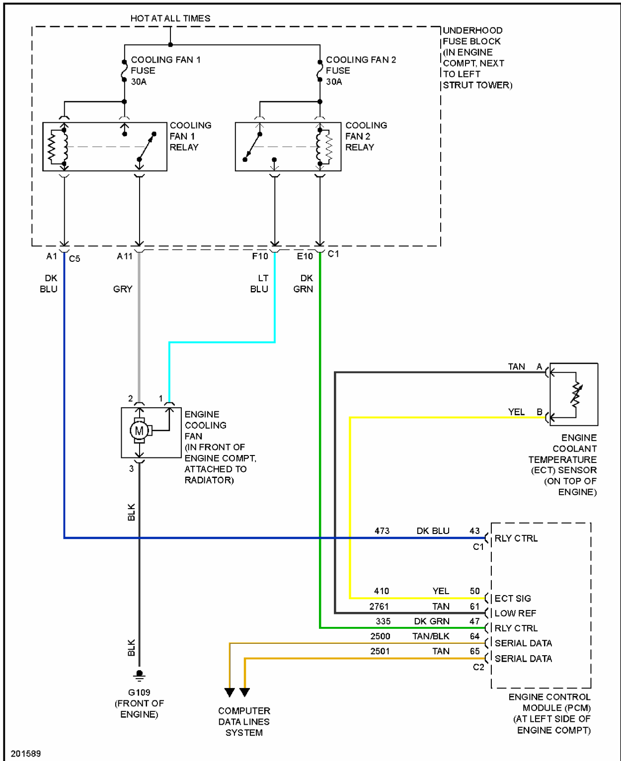
Fig. 16: 2.2L VIN F, Cooling Fan Circuit
