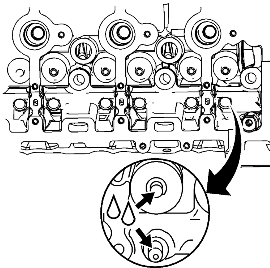
Fig. 89: Valve Tips
