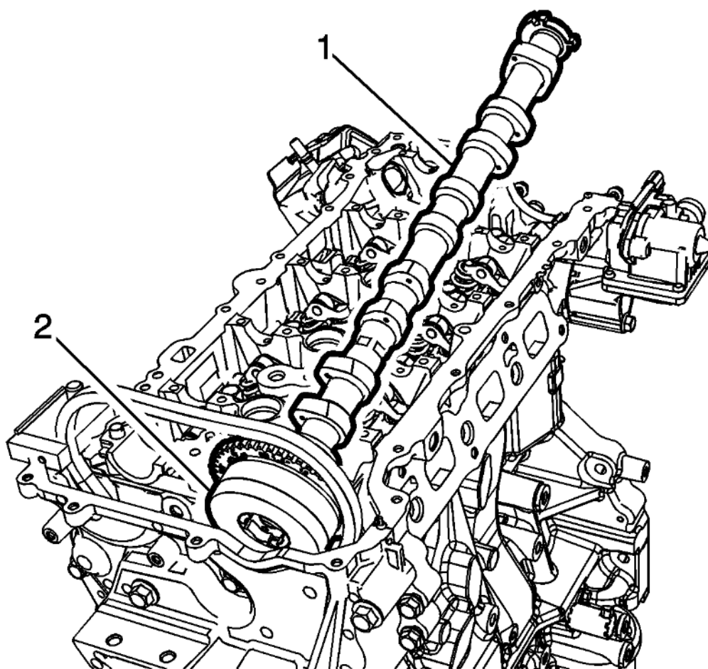
Fig. 165: Camshaft Assembly
