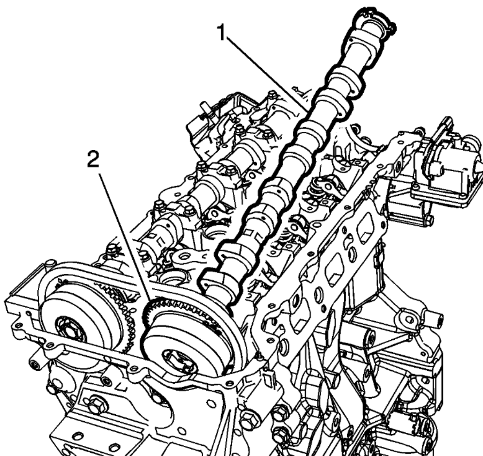
Fig. 159: Camshaft Assembly
