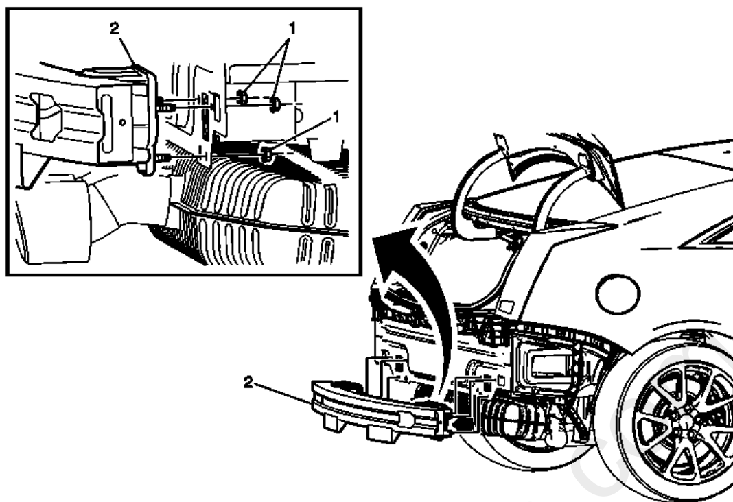
Fig. 17: Rear Bumper Impact Bar & Nuts (Coupe)
