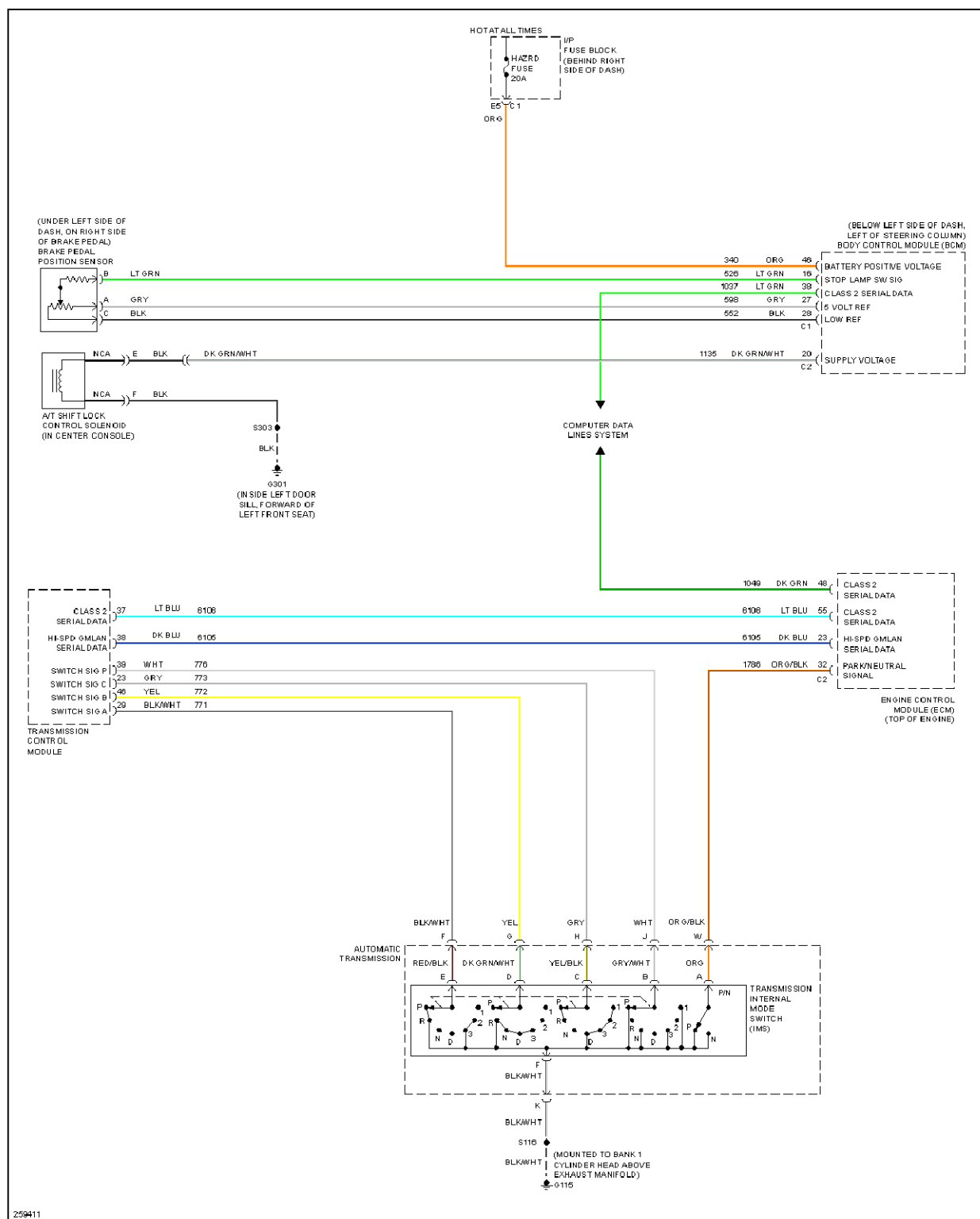
Fig. 61: 3.6L VIN 7, Shift Interlock Circuit
