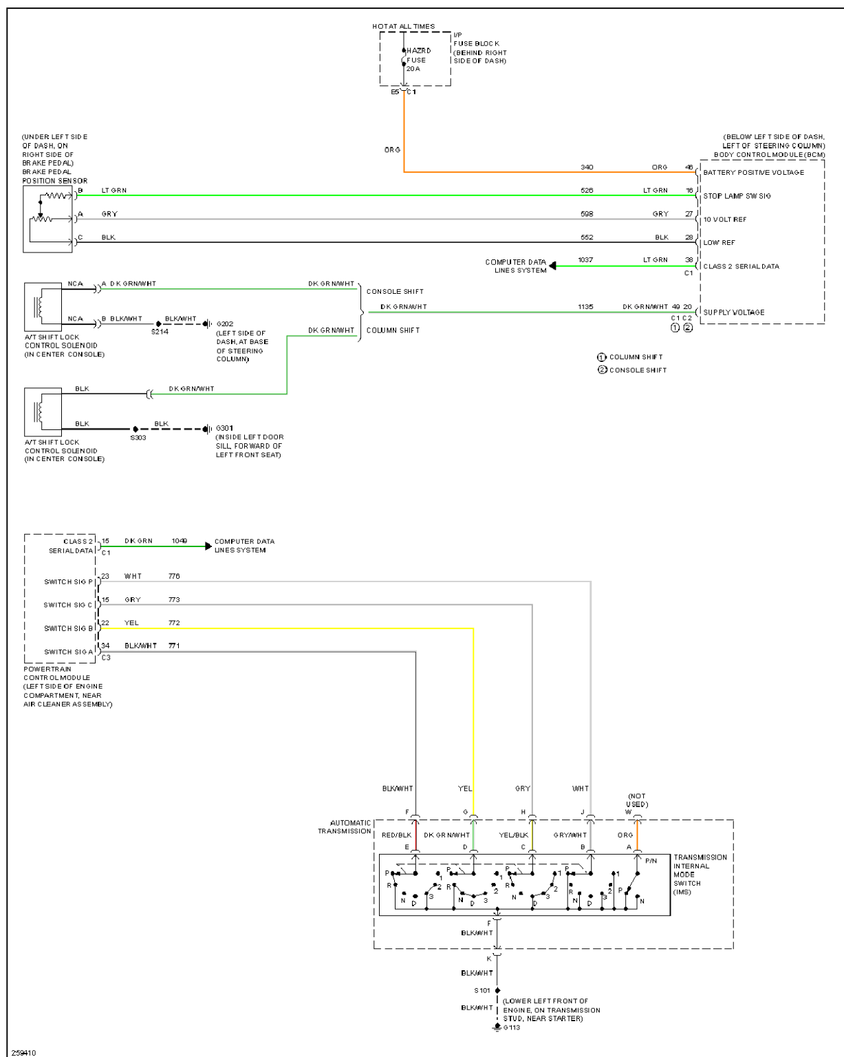
Fig. 62: 3.8L VIN 2, Shift Interlock Circuit
