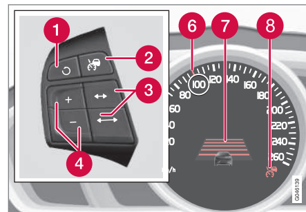
Adaptive Geschwindigkeitsregelung ohne Geschwindigkeitsbegrenzung 9 .
