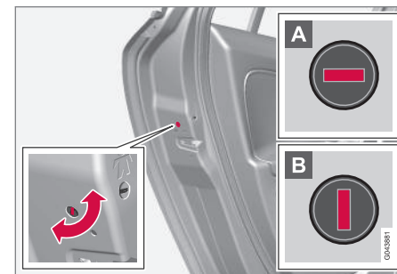
Manuelle Türverriegelung. Nicht mit der Kindersicherung (S. 191) zu verwechseln.
