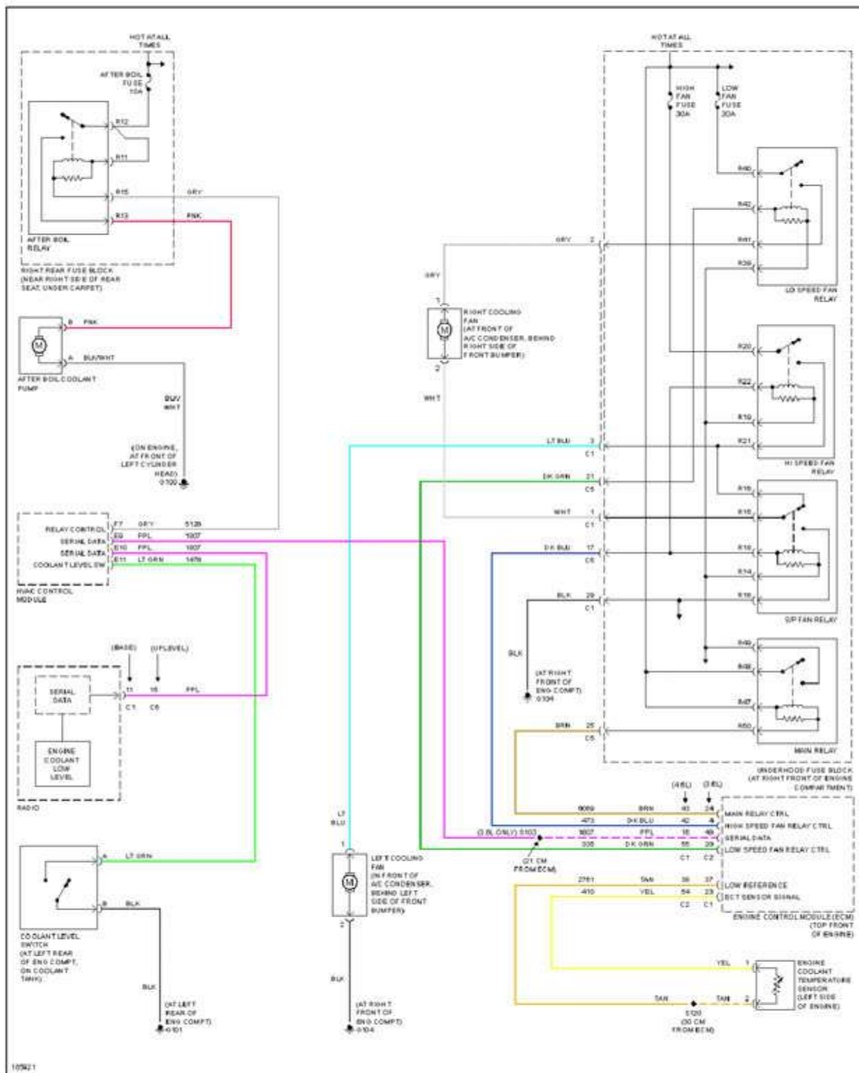
Fig. 13: Cooling Fan Circuit
