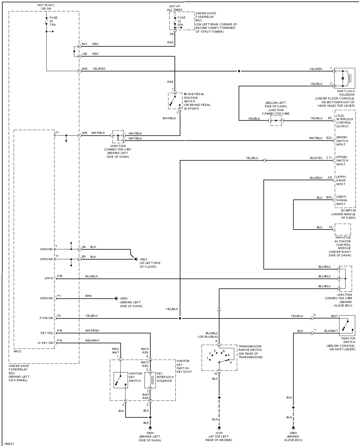
Fig. 64: Shift Interlock Circuit
