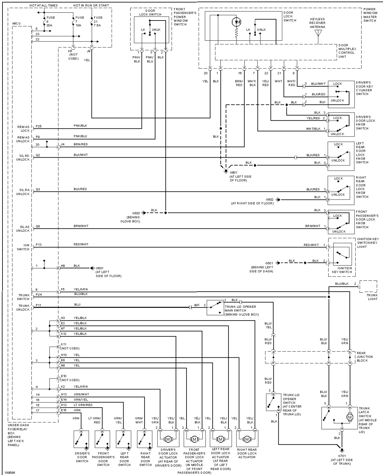
Fig. 43: Power Door Locks Circuit
