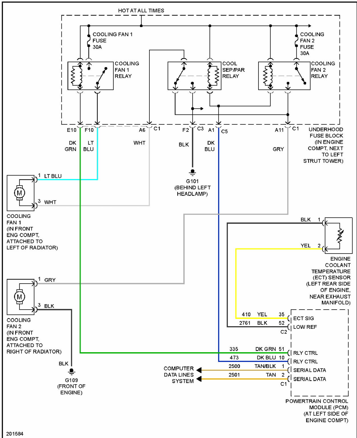
Fig. 15: 2.0L VIN P, Cooling Fan Circuit
