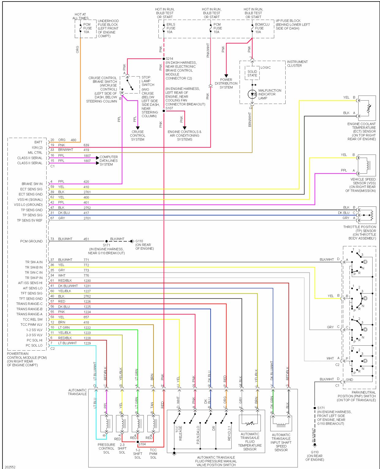
Fig. 39: A/T Circuit
