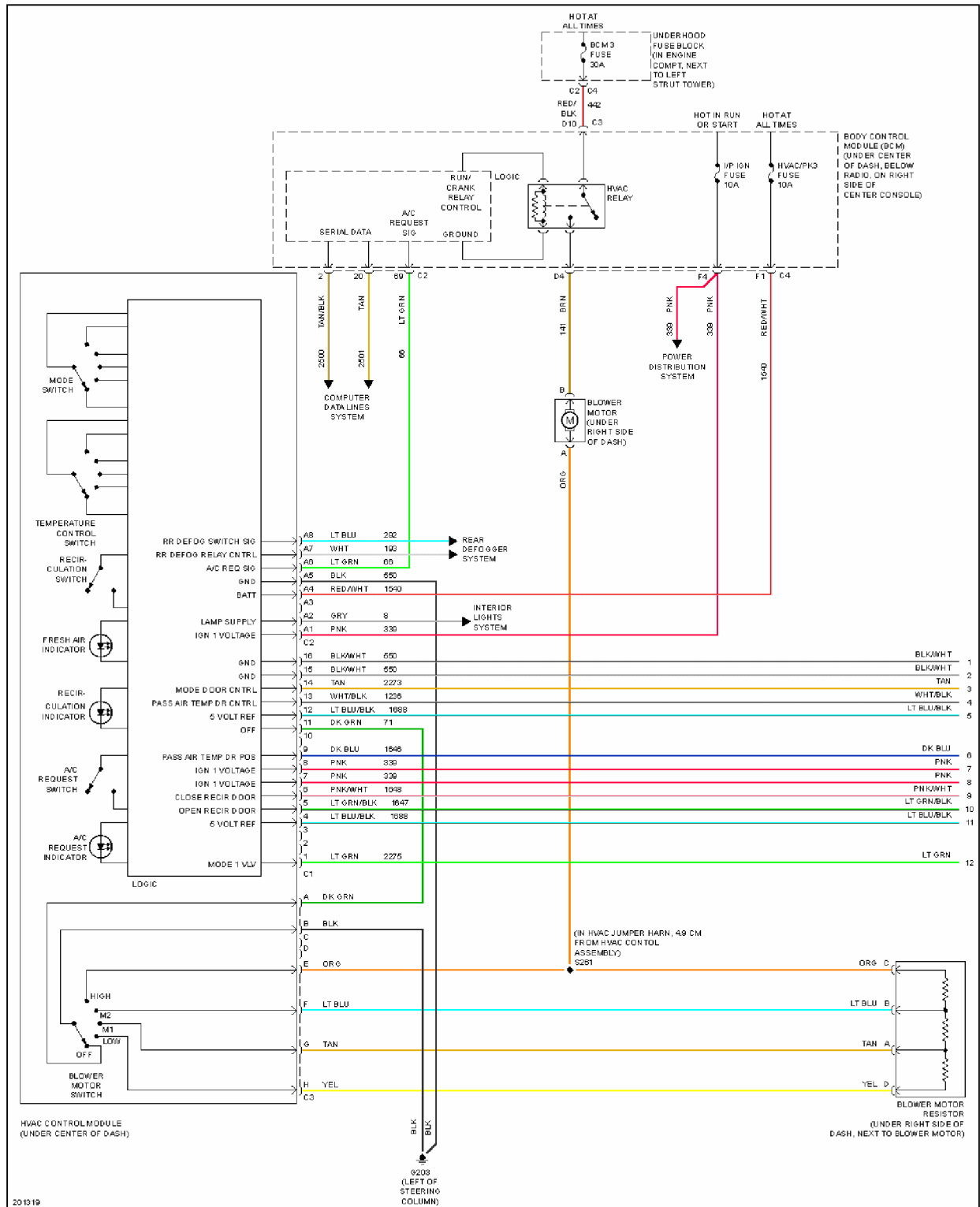
Fig. 2: 2.0L VIN P, Manual A/C Circuit (1 of 2)
