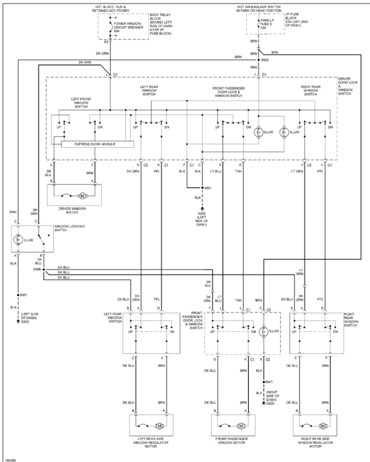
Fig. 46: Power Window Circuit, 4 Door
