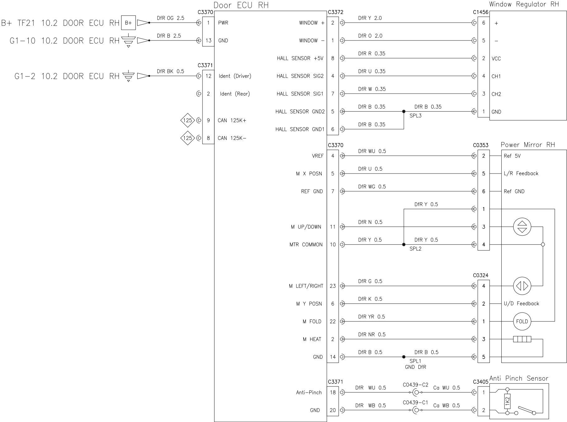
Door-Front Right LHD (Passenger Door Switchpack)
