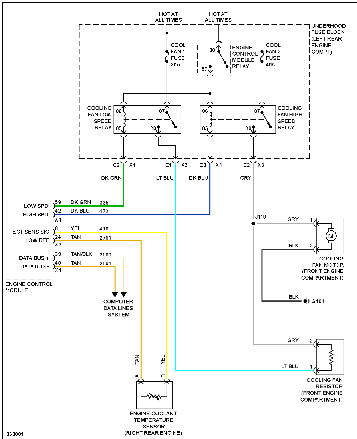
Fig. 14: 2.4L VIN W, Cooling Fan Circuit
