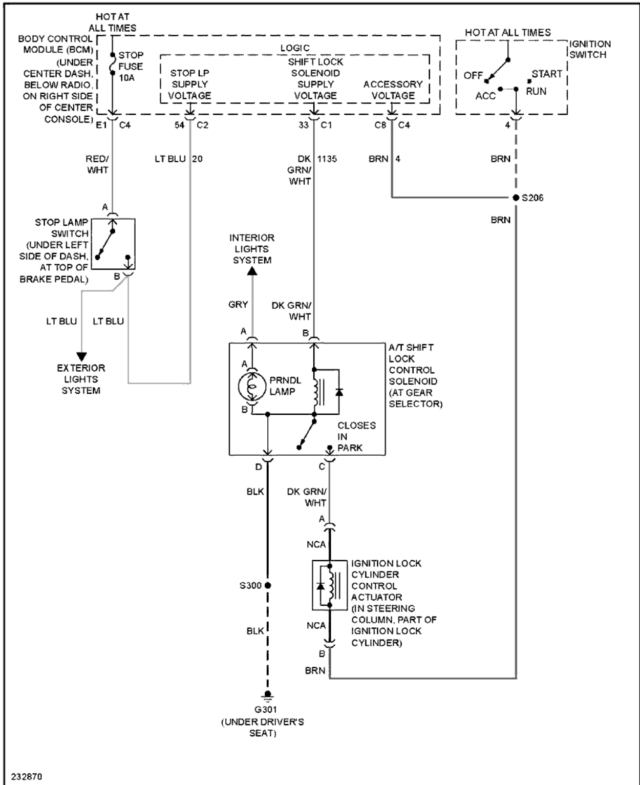
Fig. 48: Shift Interlock Circuit
