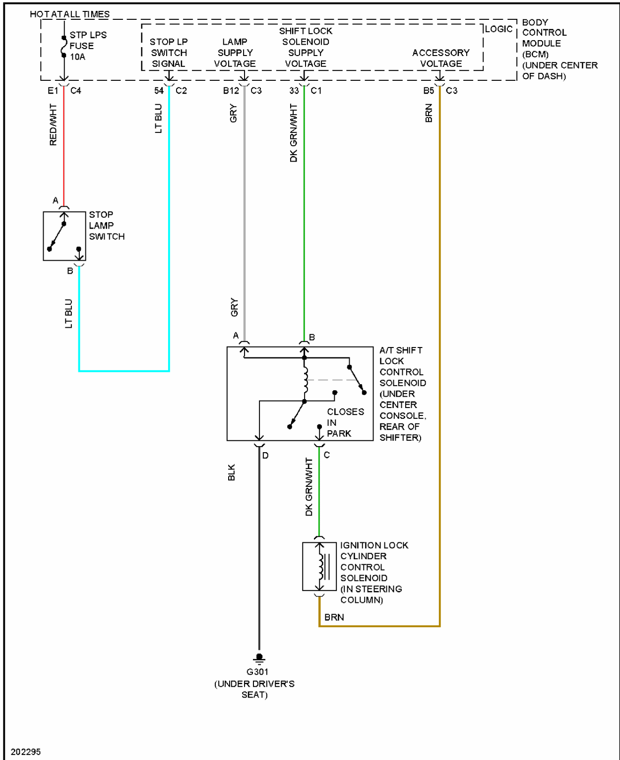
Fig. 53: Shift Interlock Circuit
