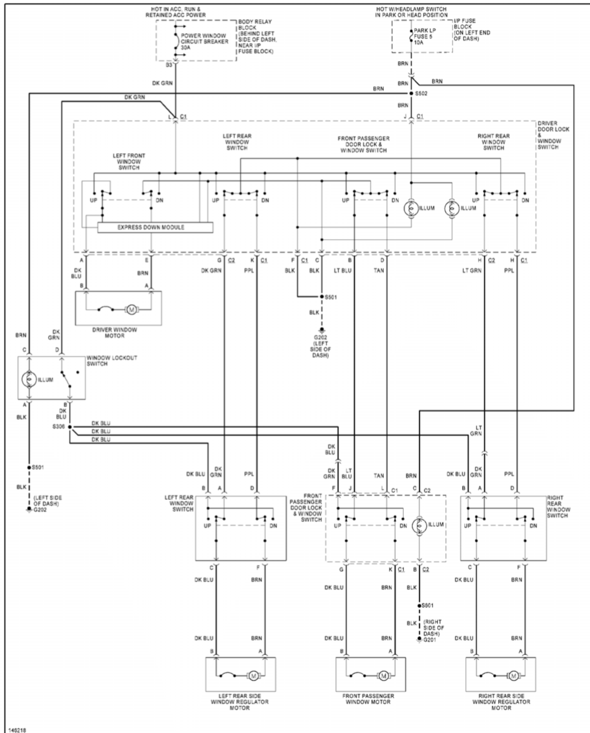
Fig. 47: Power Window Circuit, 4 Door
