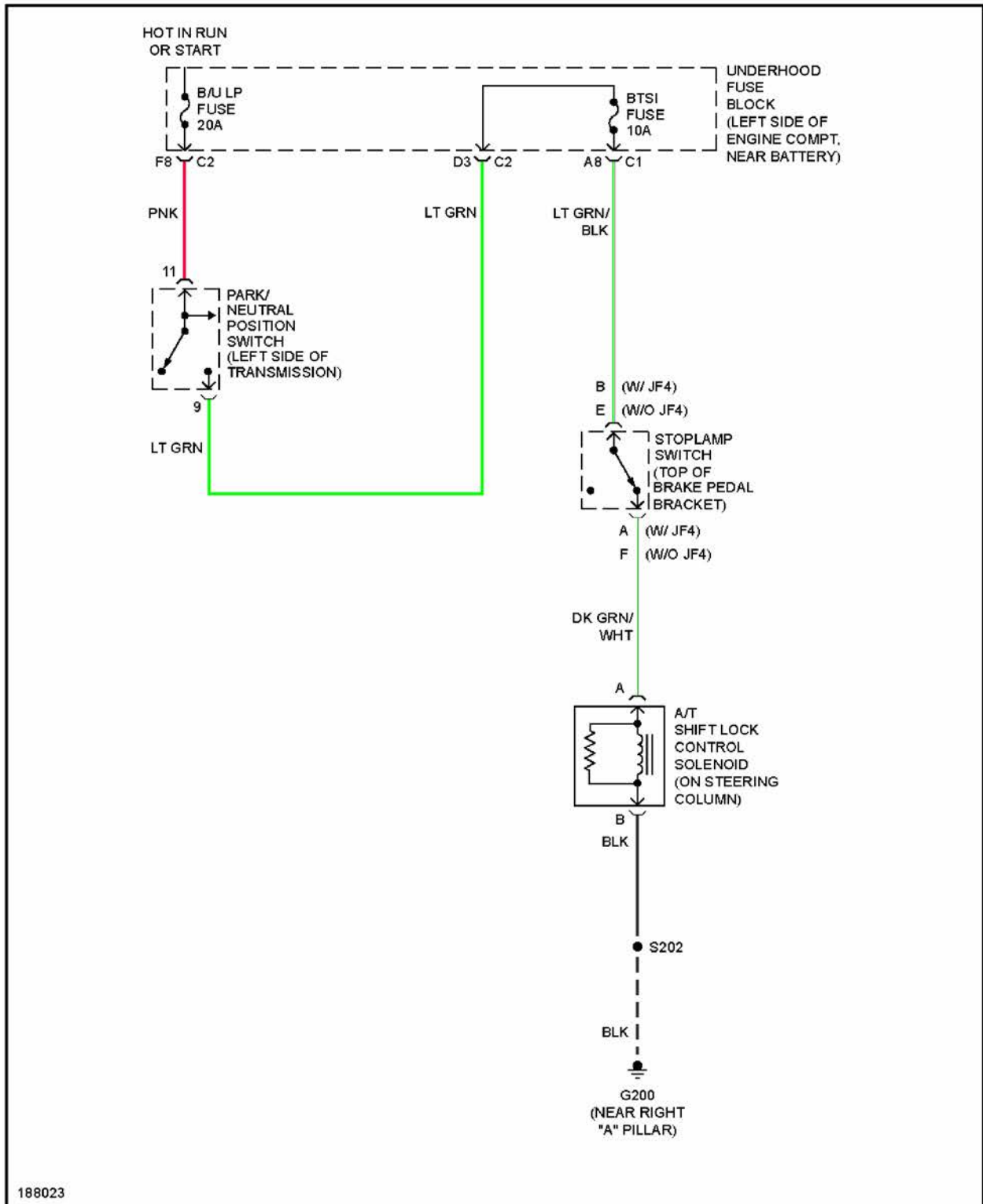
Fig. 87: Shift Interlock Circuit
