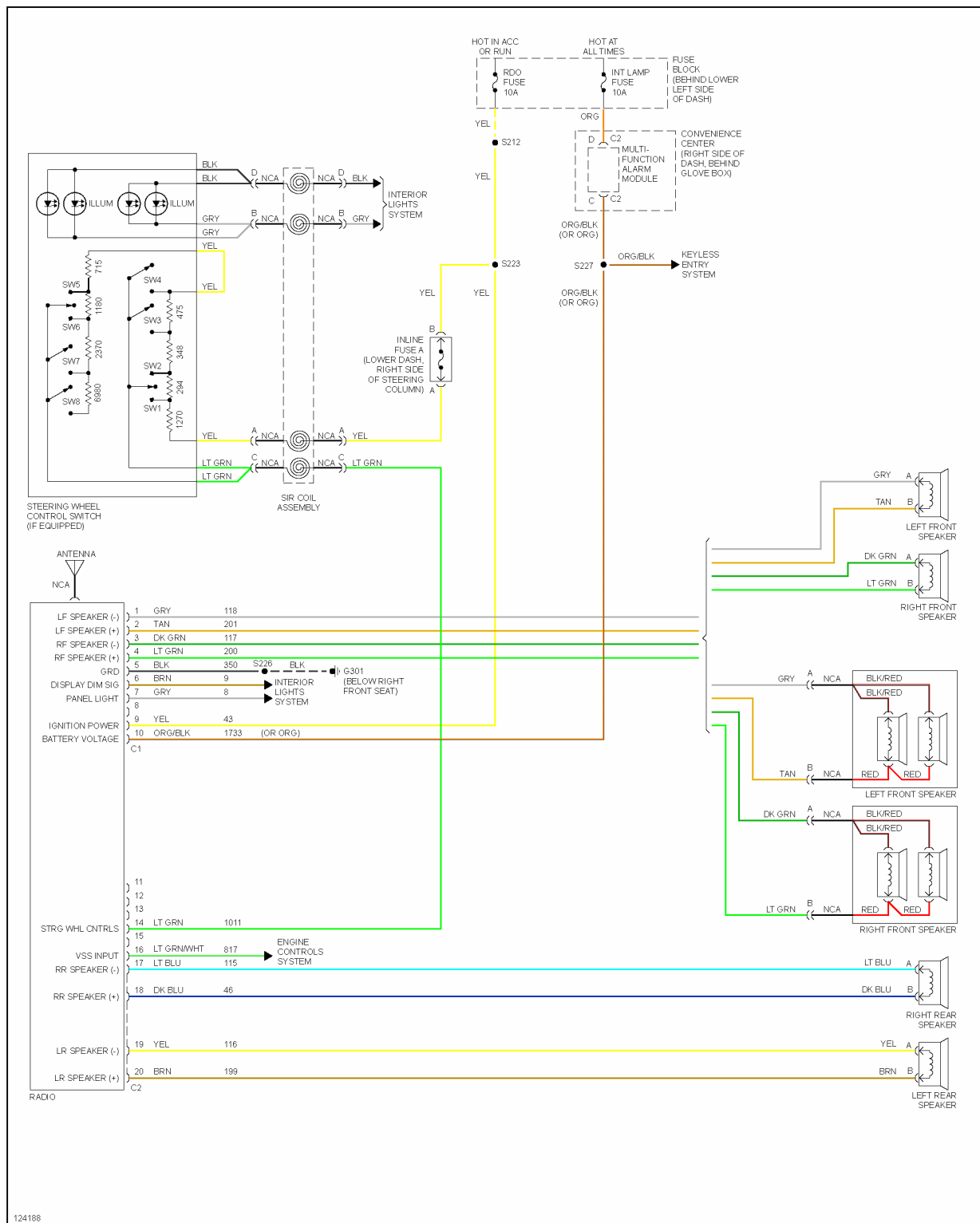
Fig. 38: Radio Circuits
