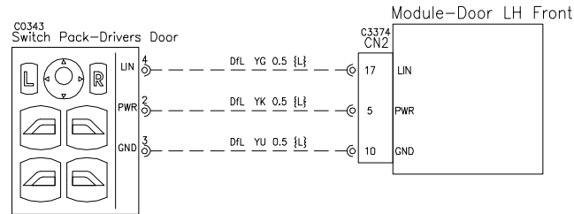
Door-Front Left LHD (Driver Door Switchpack)
