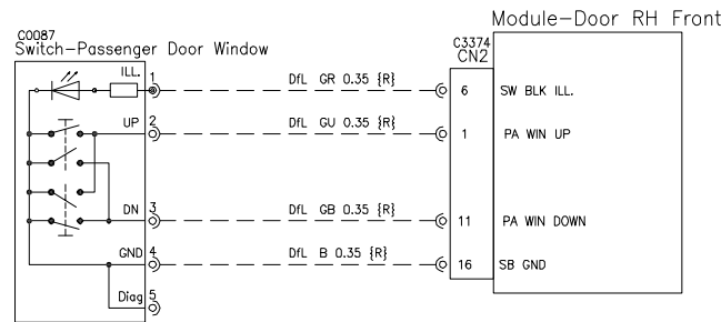
Door-Front Left RHD (Passenger Door Switchpack)
