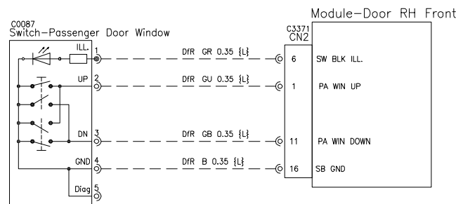
Door-Front Right LHD (Passenger Door Switchpack)
