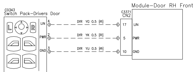
Door-Front Right RHD (Driver Door Switchpack)
