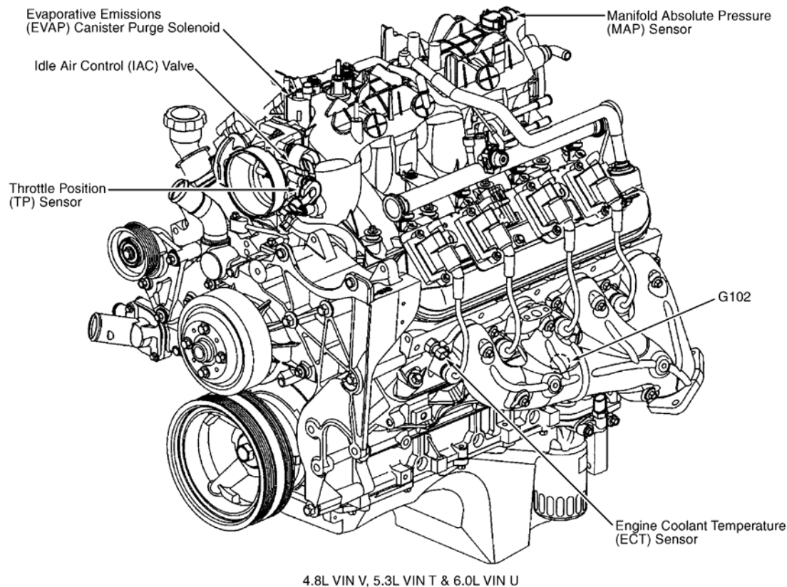
Fig. 5: Left Side Of Engine (4.8L VIN V, 5.3L VIN T & 6.0L VIN U) Courtesy of GENERAL MOTORS CORP.
