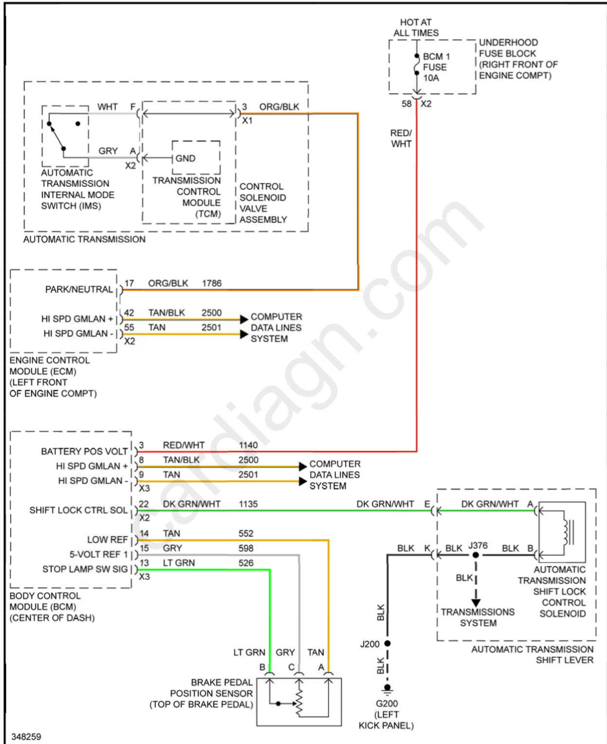
Fig. 110: Shift Interlock Circuit
