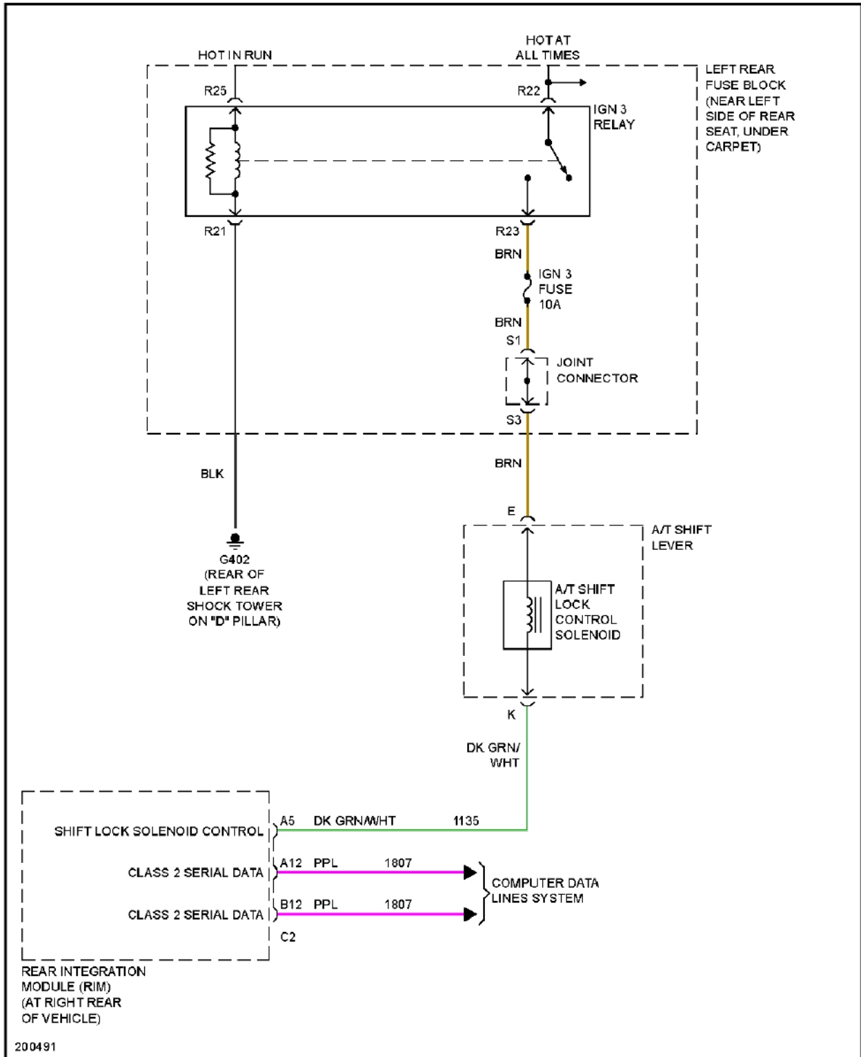
Fig. 78: Shift Interlock Circuit
