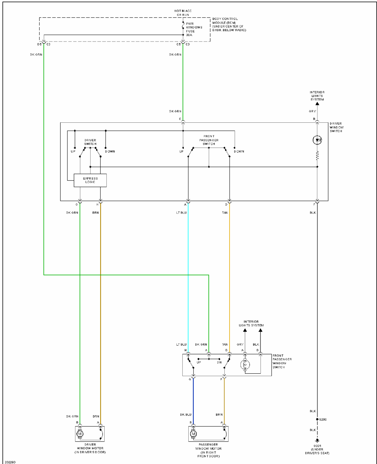
Fig. 48: Power Windows Circuit, Coupe
