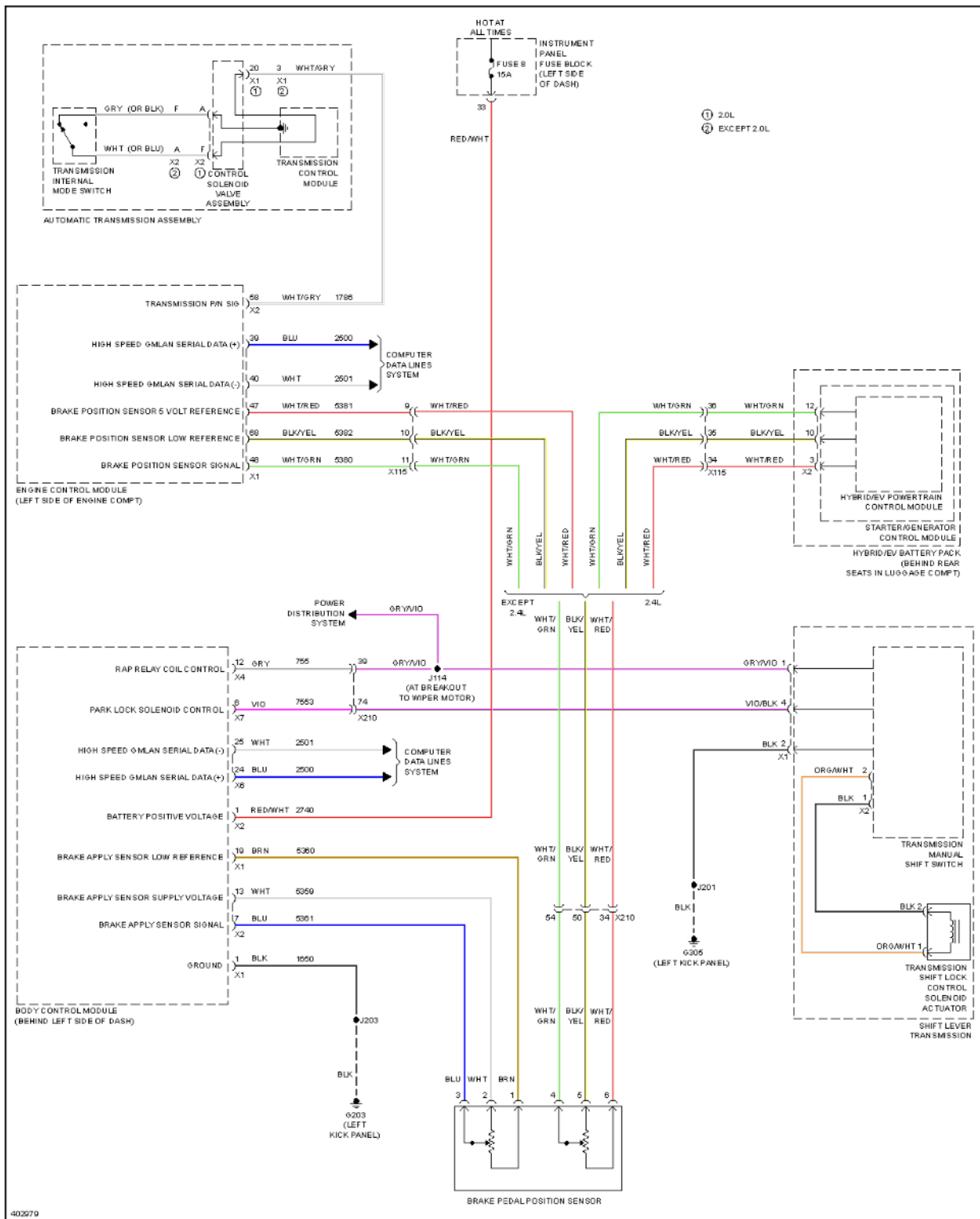
Fig. 123: Shift Interlock Circuit
